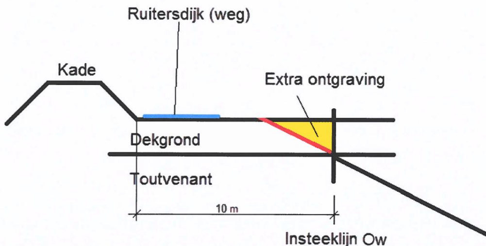
Afbeelding 1 – schematische weergave extra ontgraving
