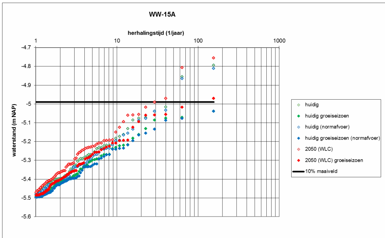
Figuur 4.3 Waterstandkansgrafieken peilvak WW-15A
