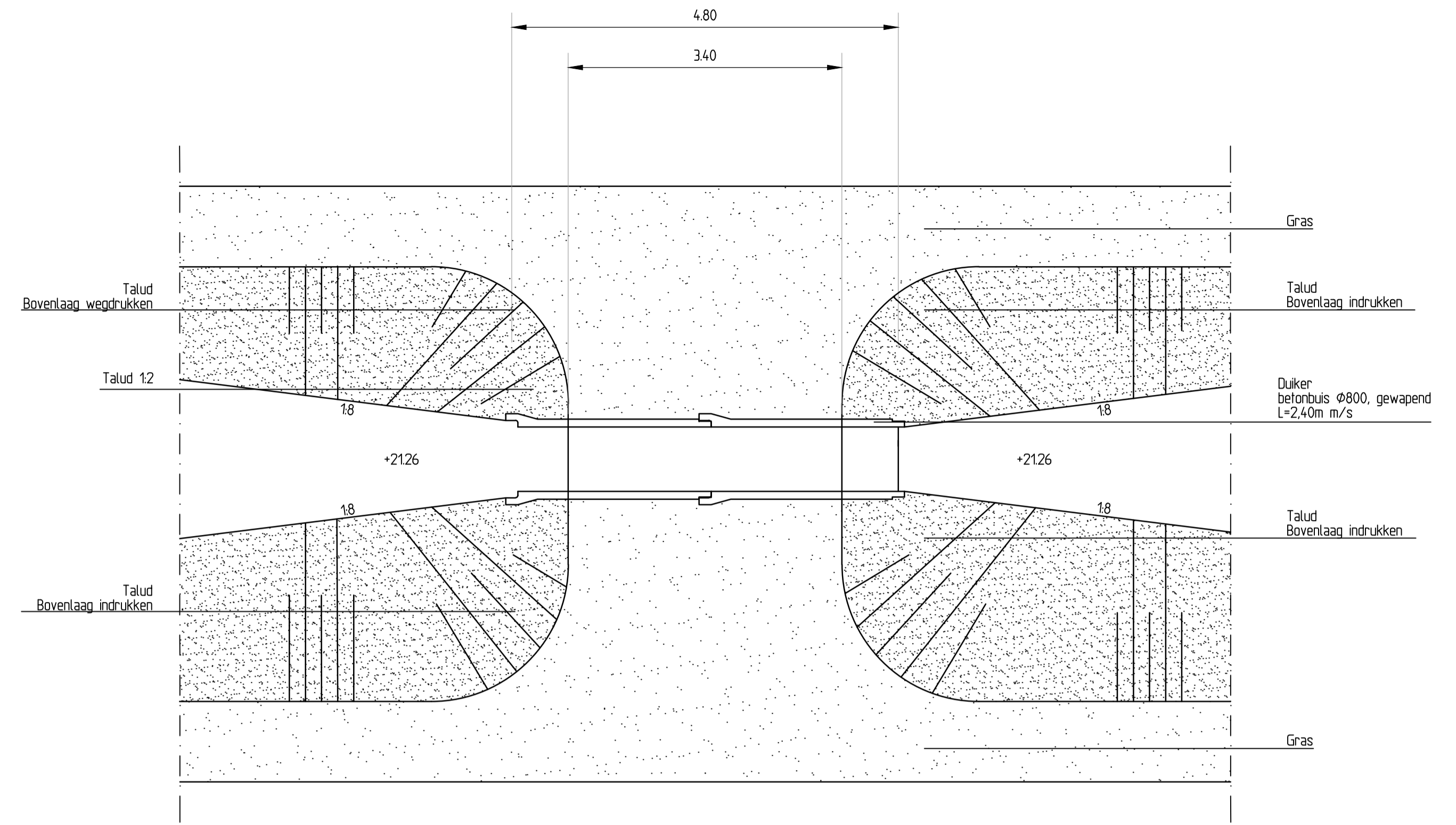
Bovenaanzicht duiker schaal: 1 : 50
