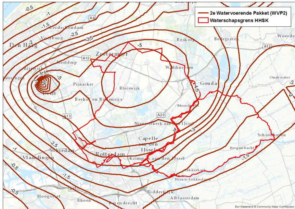
Figuur 0-16: Isohyphenpatroon WVP2, TNO 28-4-1995
