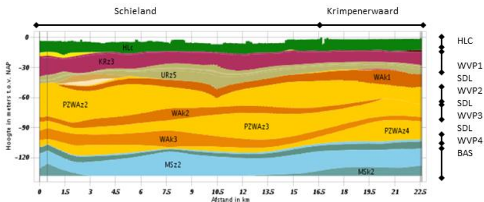
Figuur 3-4: Dwarsdoorsnede bodemopbouw REGIS II noord-zuid, Zoetermeer tot Lekkerkerk
