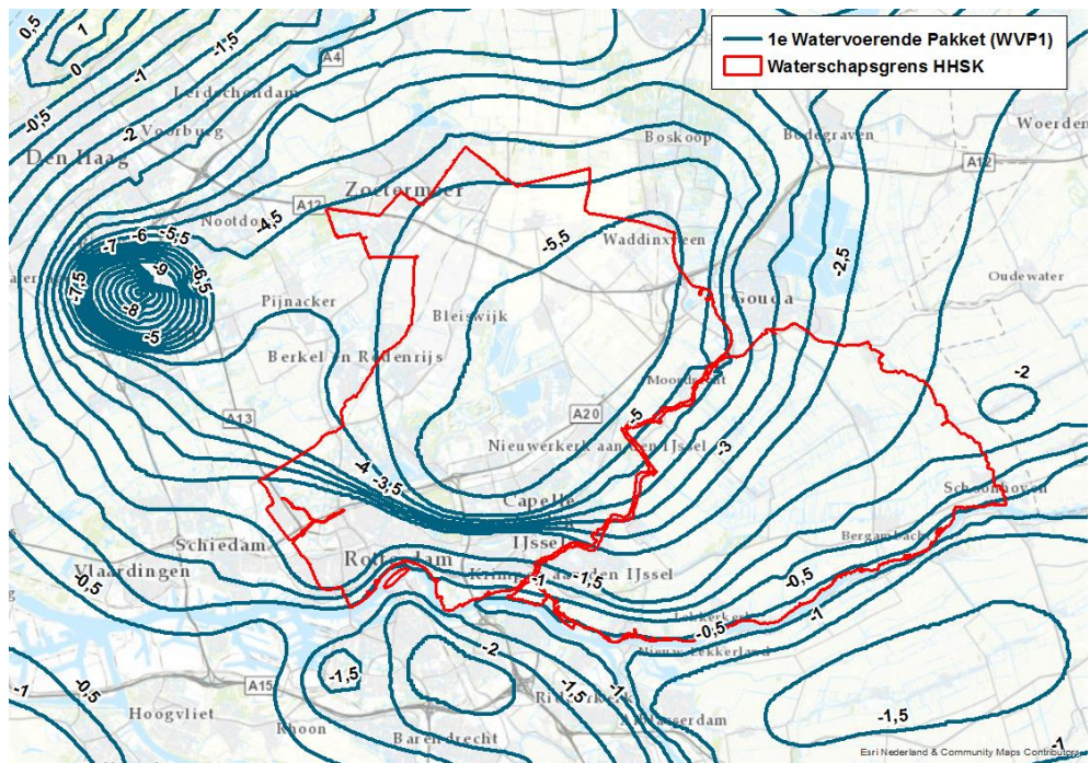
Figuur 0-14: Isohypsenvoerpatroon WVP1, TNO 28-4-1995
