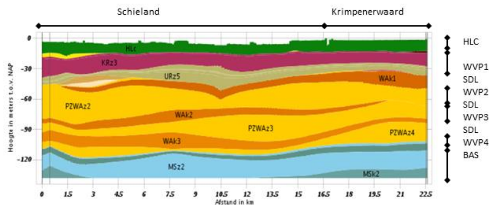
Figuur 0-5: Dwarsdoorsnede bodemopbouw REGIS II v2.2 oost-west, N471 tot Schoonhoven
