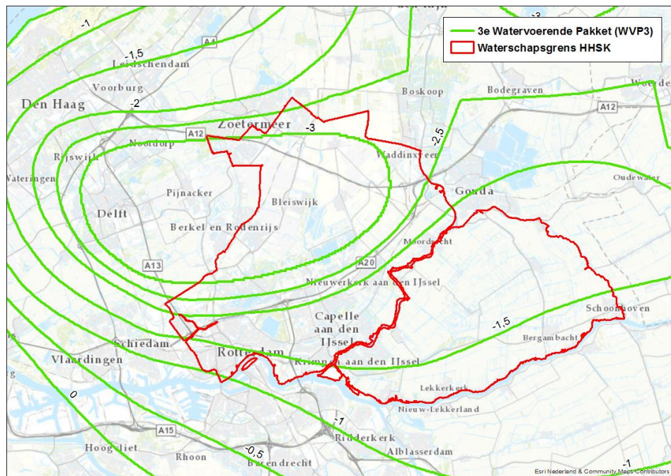
Figuur 0-17: Isohyphenpatroon WVP3, TNO 28-4-1995
