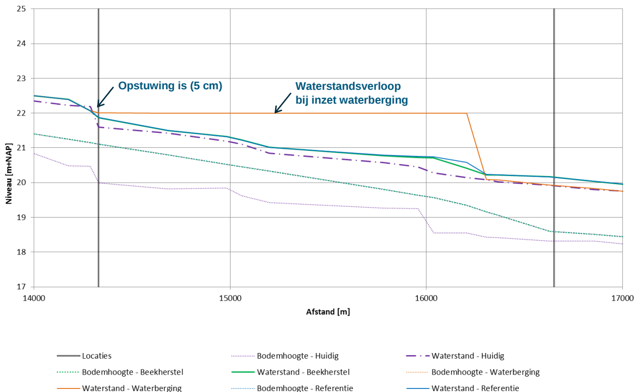
Figuur 6.5 Lengteprofiel berekende waterstanden T100Wh waterbergingsgebied
