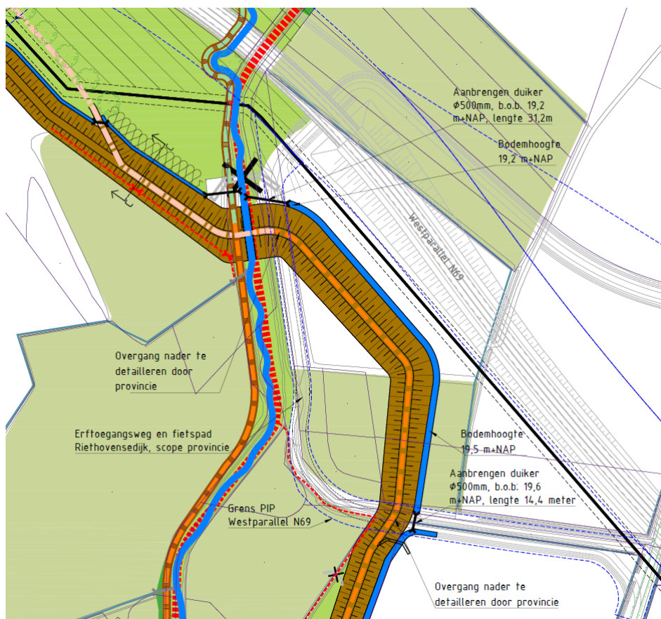
Figuur 3.4: Variant kade
