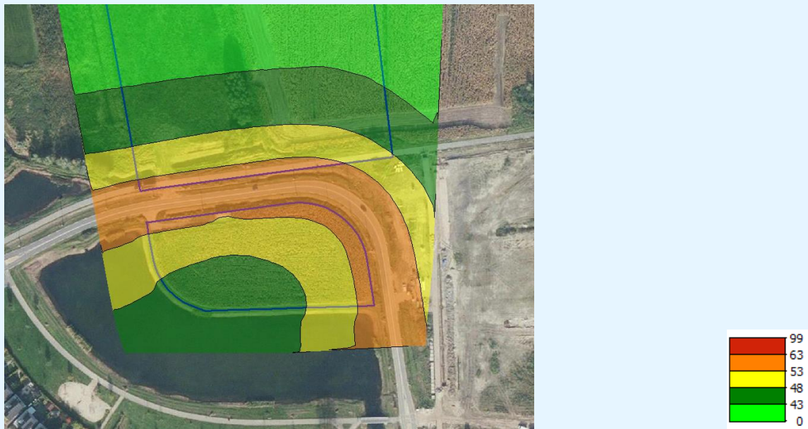
figuur 3: geluidscontouren wegverkeer door de Minervasingel (op 5m boven maaiveld, na aftrek van 5 dB)
