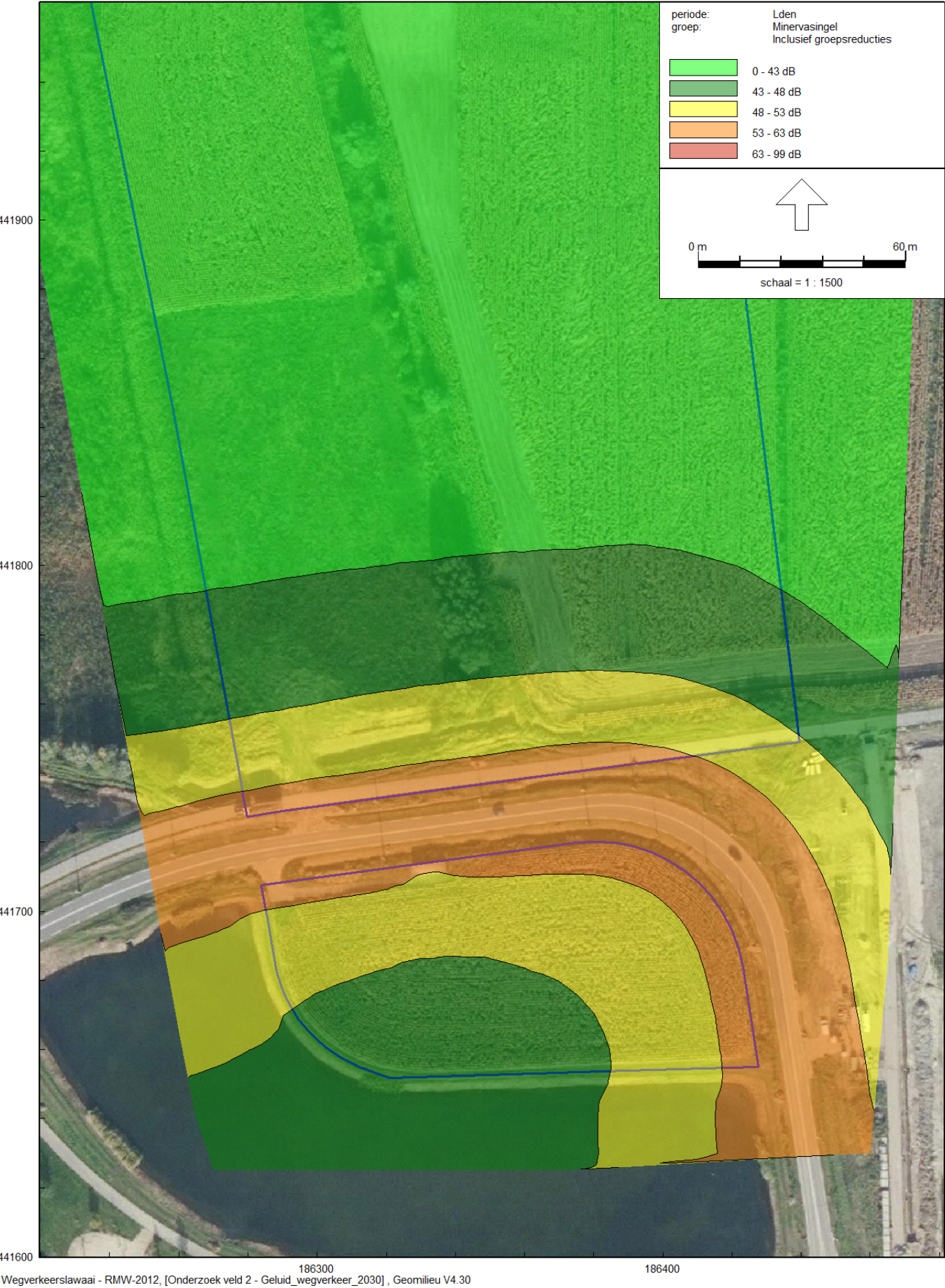
Geluidcontouren Minervasingel (rekenhoogte 5 meter), na aftrek van 5 dB conform artikel 110g Wgh
