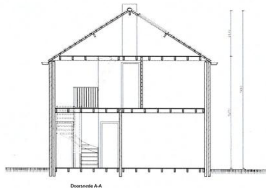
doorsnede van jaren '50/'60 woning
