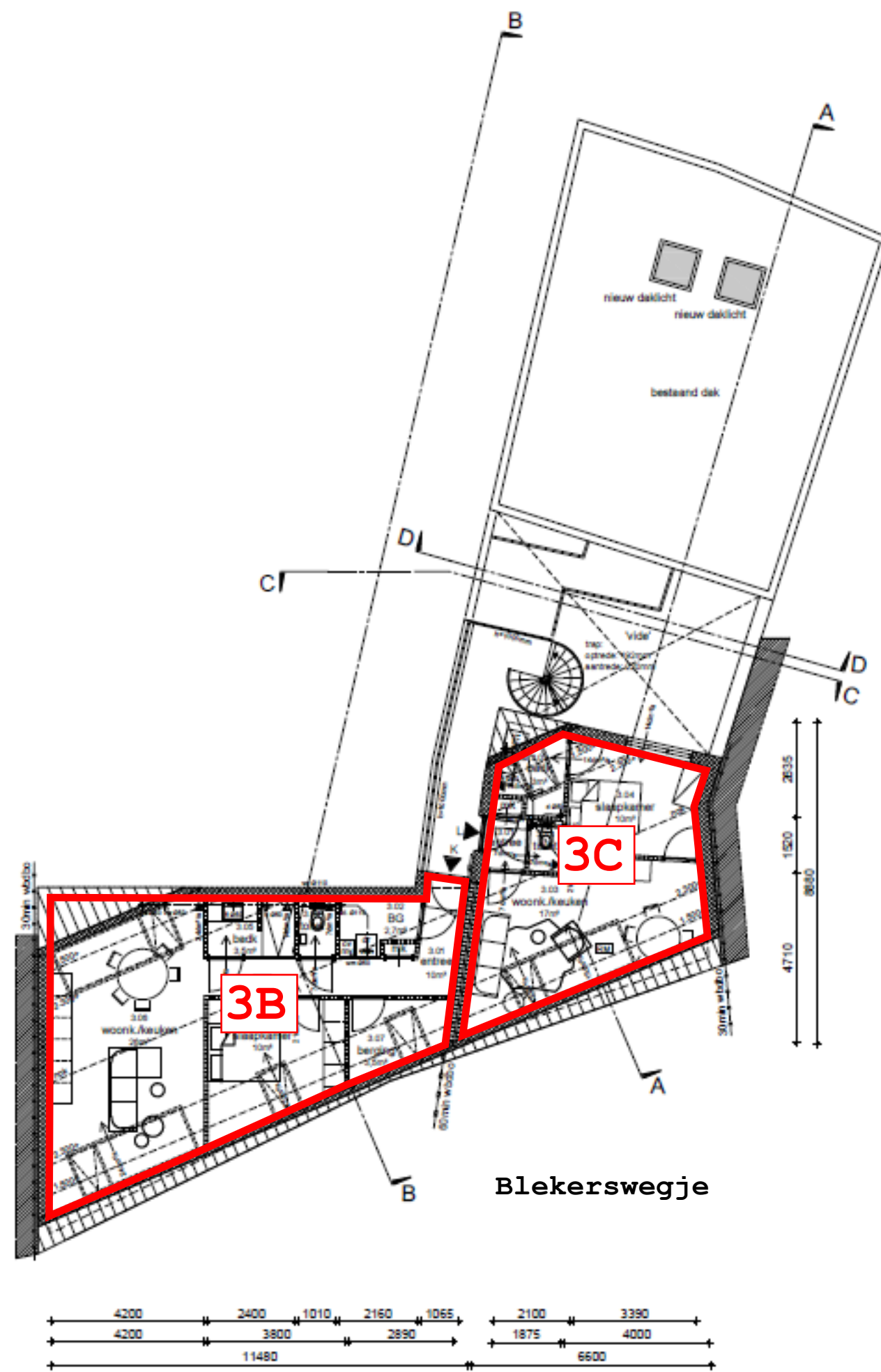
3e verdieping
