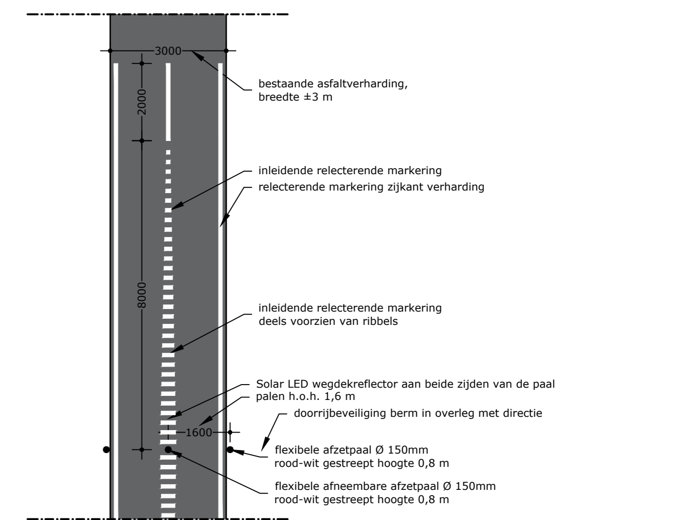
PRINCIPEDETAIL 1: PAAL OP HET FIETSPAD Schaal 1:100
