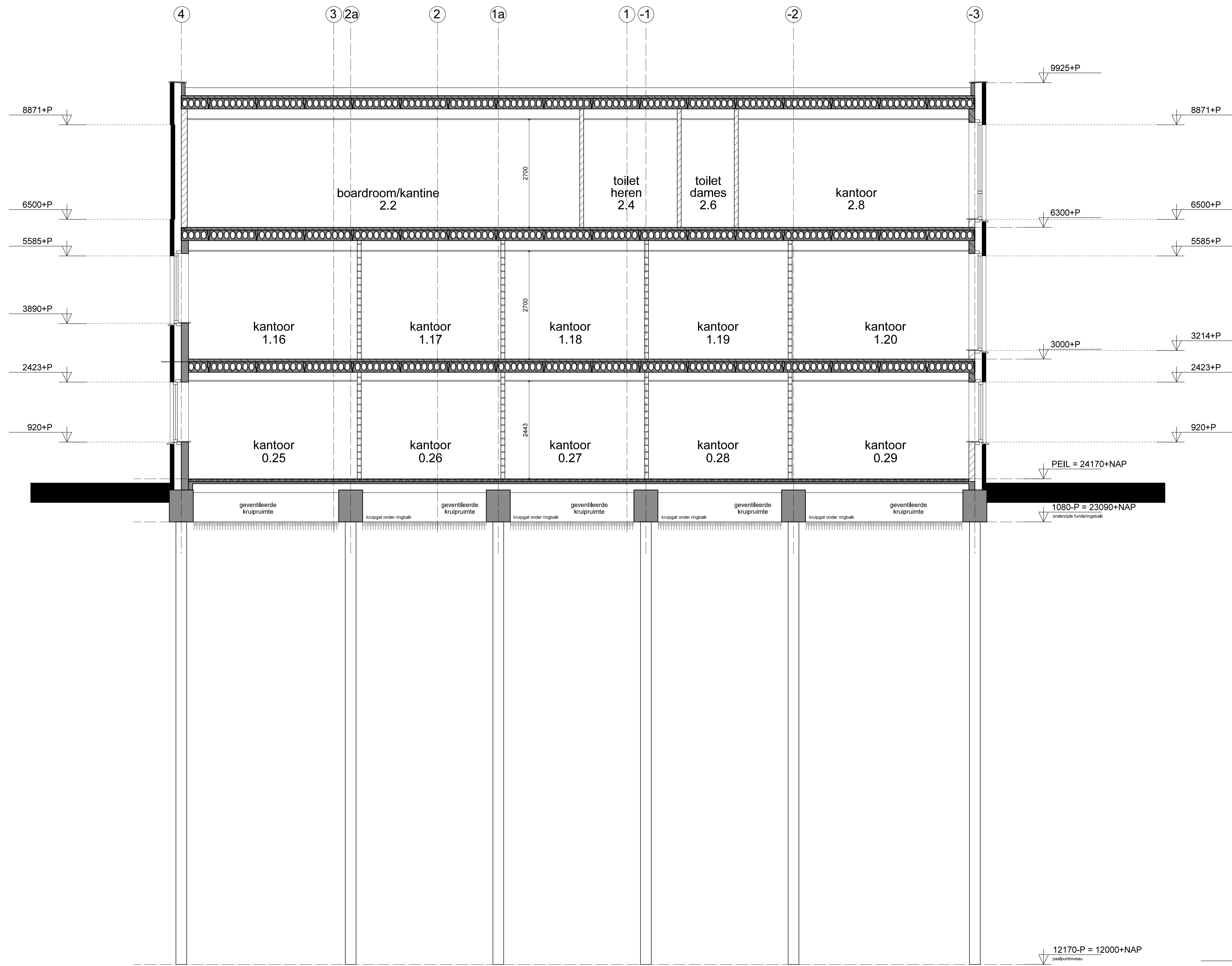
DOORSNEDE A-A
