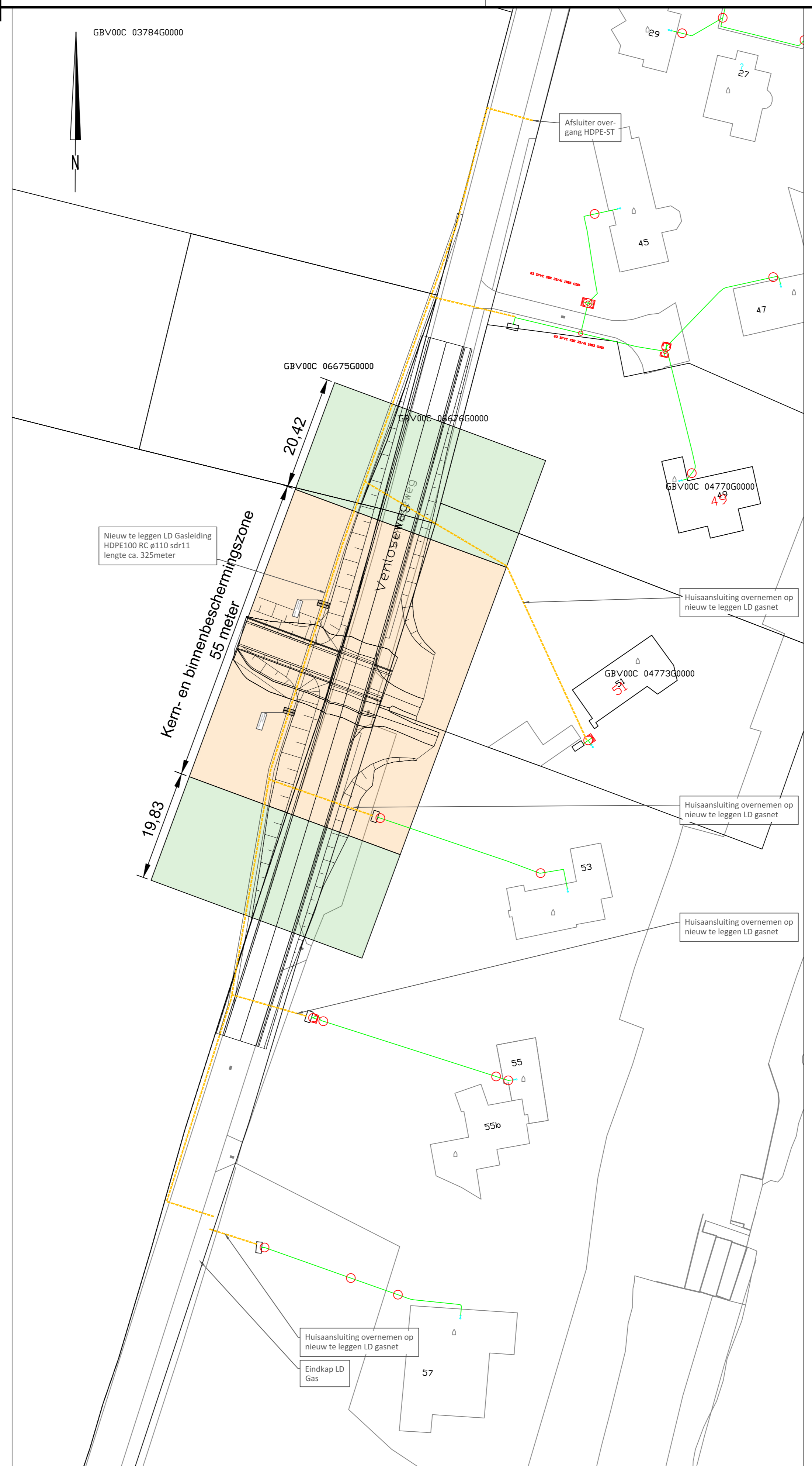
Aanpassingen Lagedruk Gas Schaal 1:100
