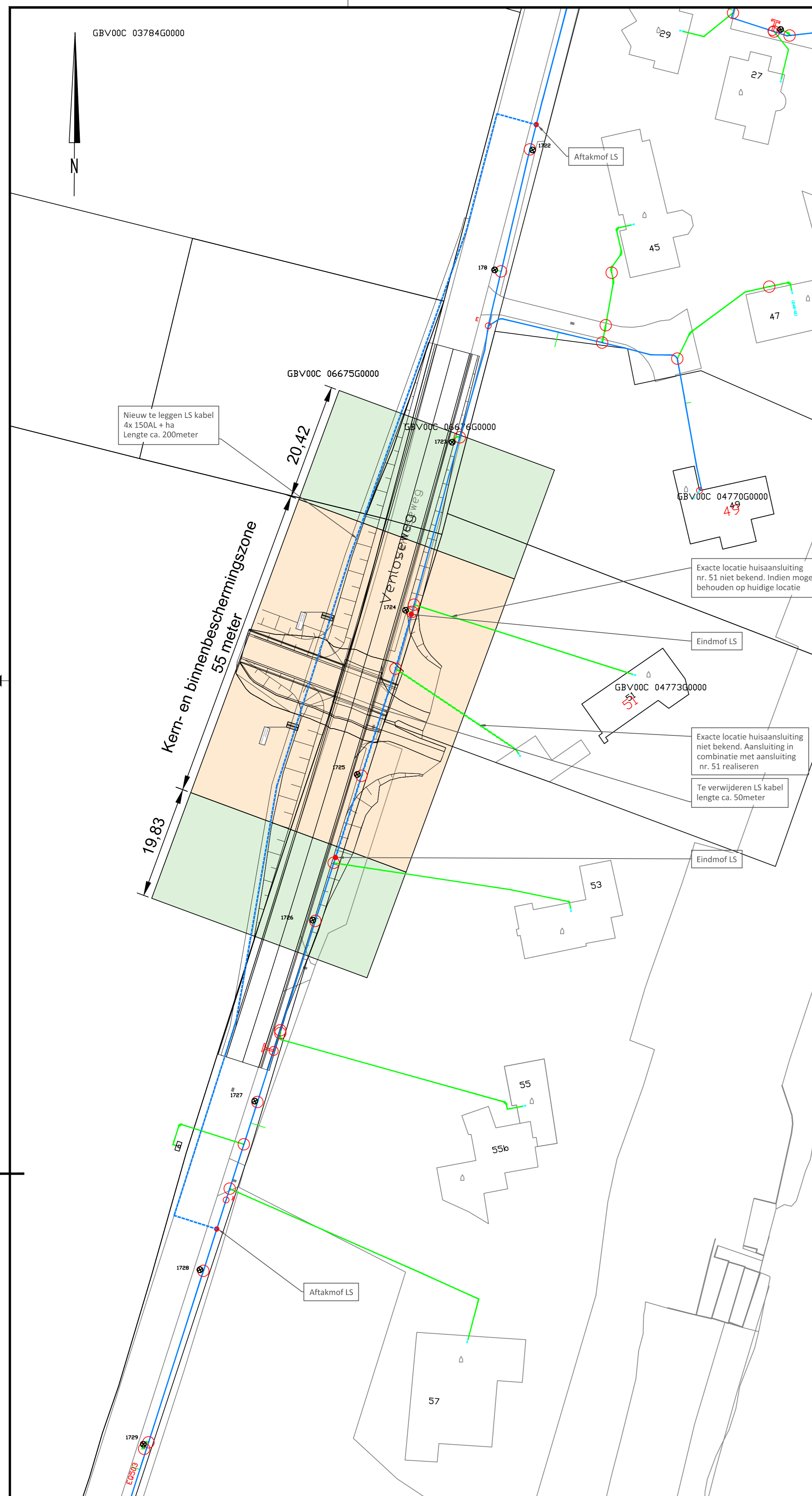
Aanpassingen Laagspanning Schaal 1:100
