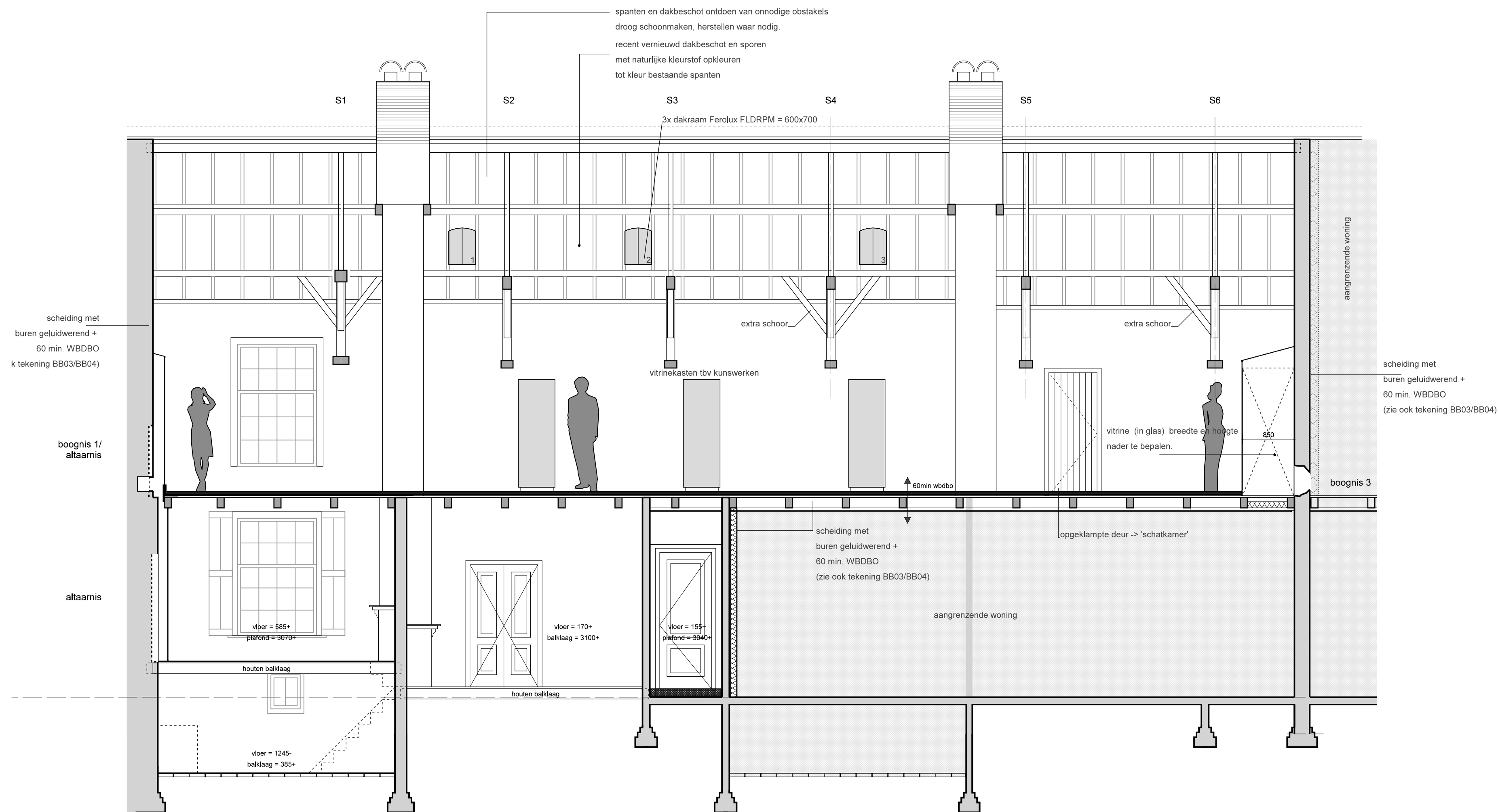
principeddoorsnede C
