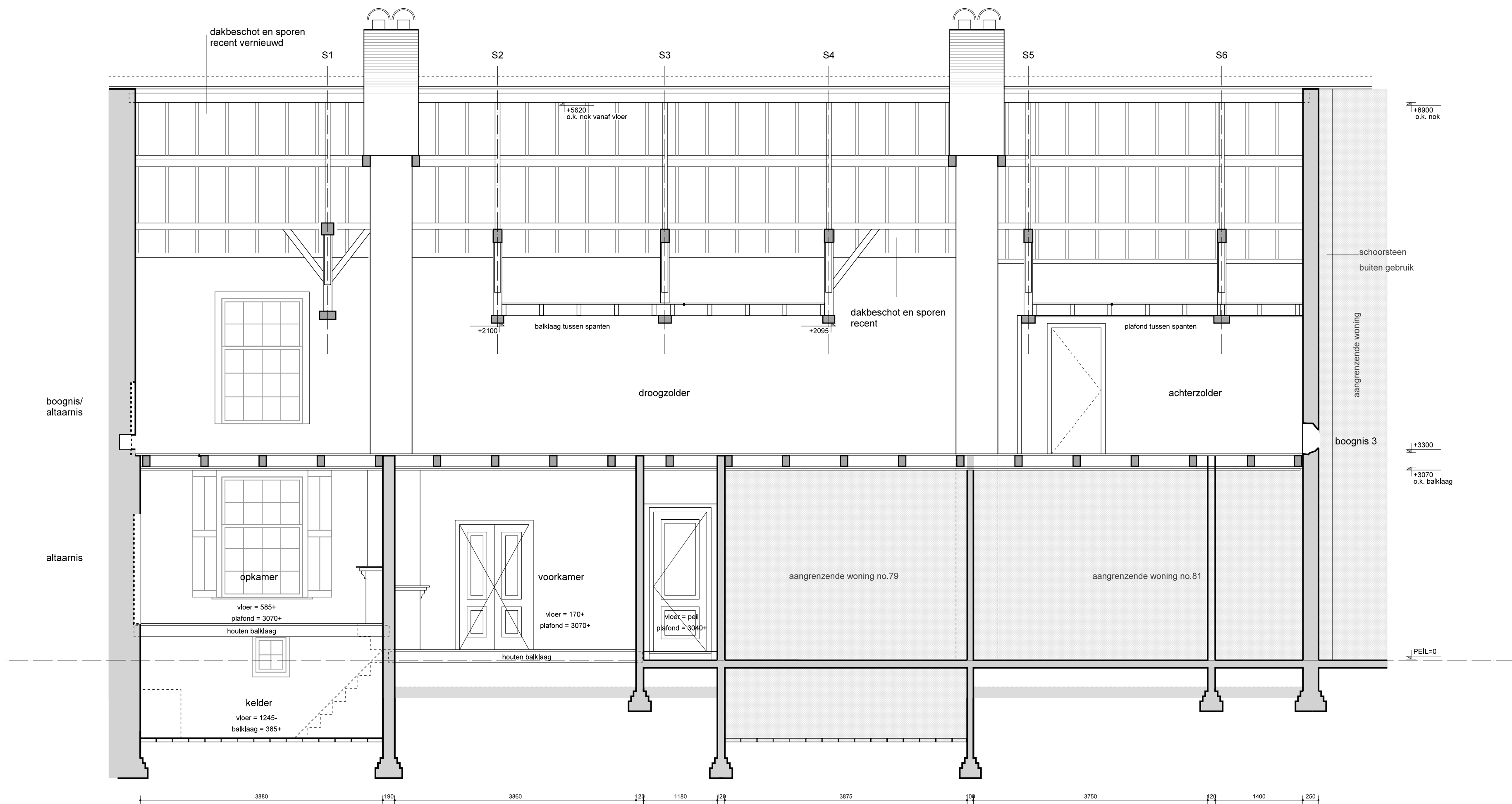
principeddoorsnede C
