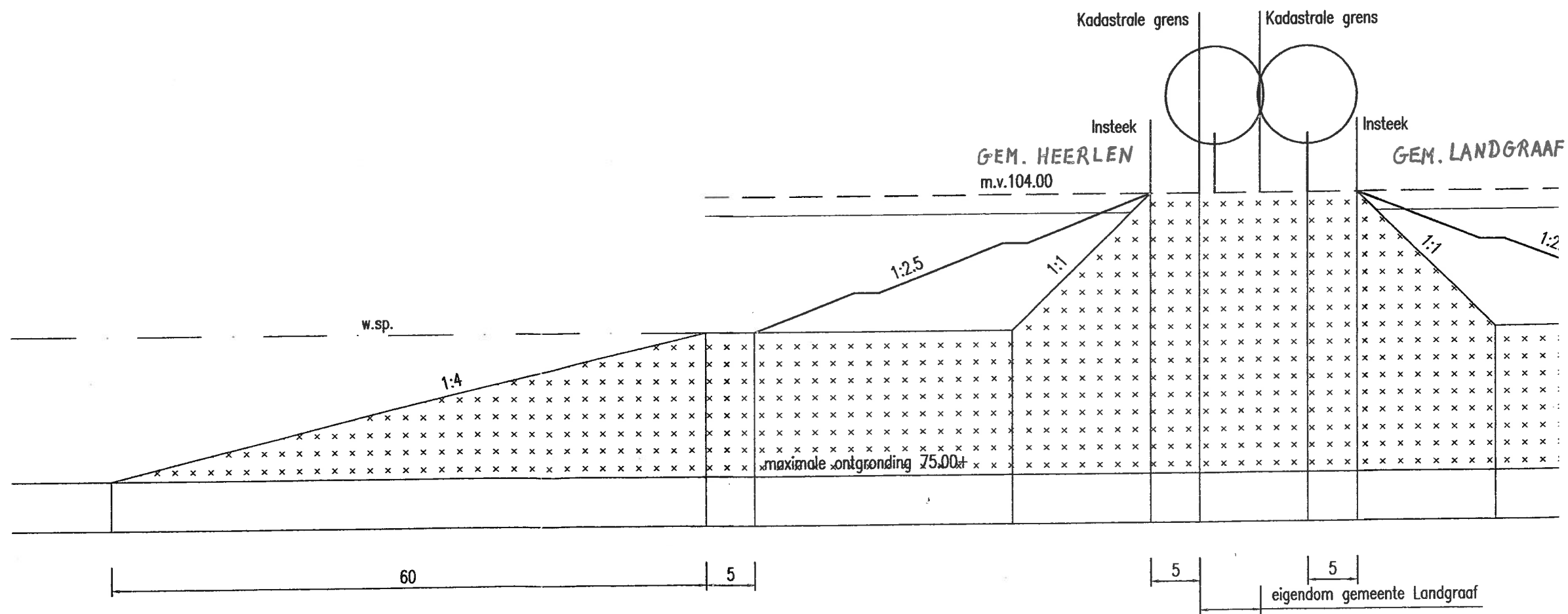
NORMPROFIEL, Schaal 1:500
