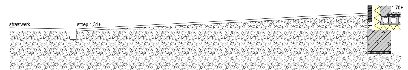
hoogtedoorsnede A
