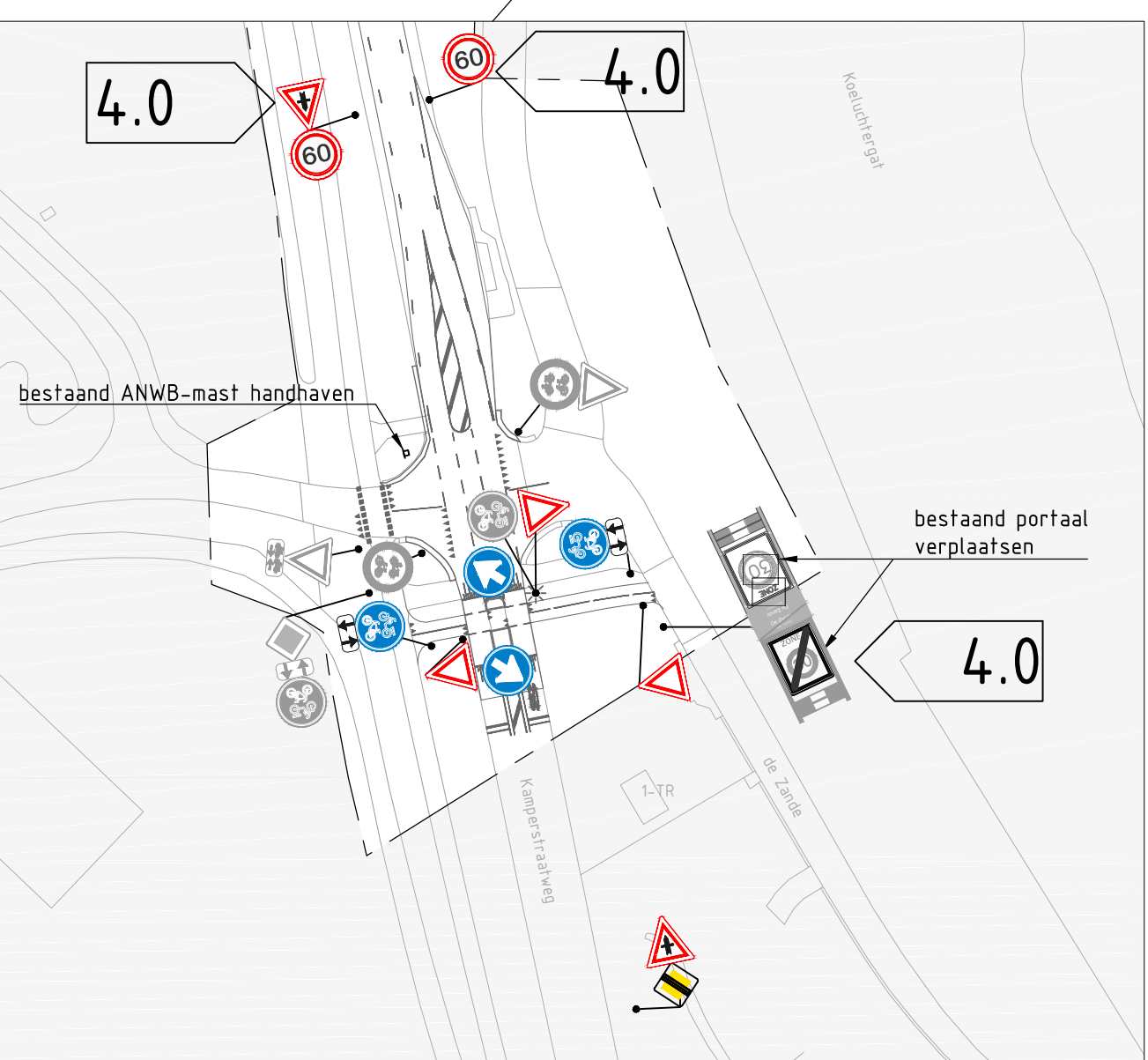
Kruising Jules van Hasseltweg/Kamperstraatweg
