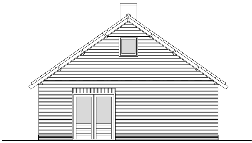
OOSTGEVEL
