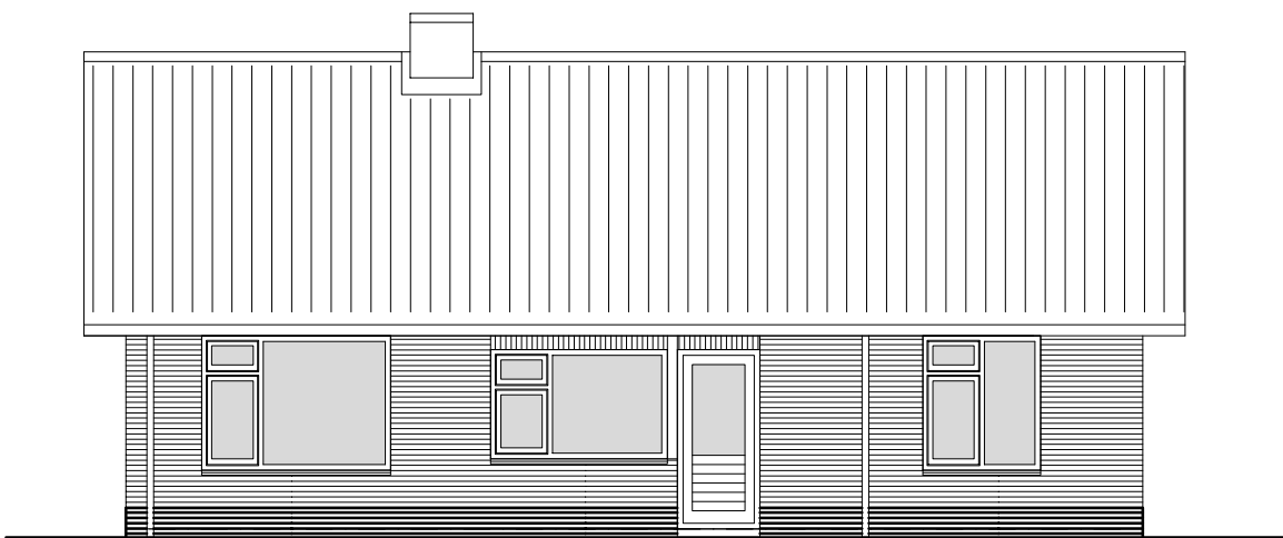
ZUIDGEVEL
