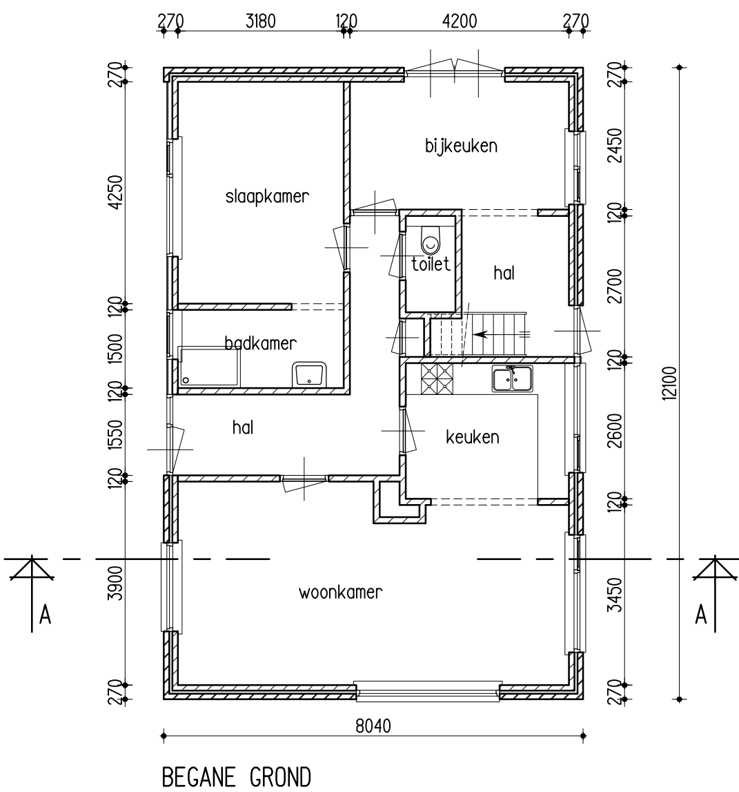
BEGANE GROND
