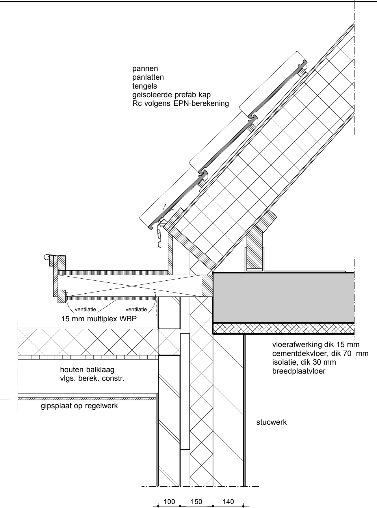
aansluiting platdak / gevel met goot
