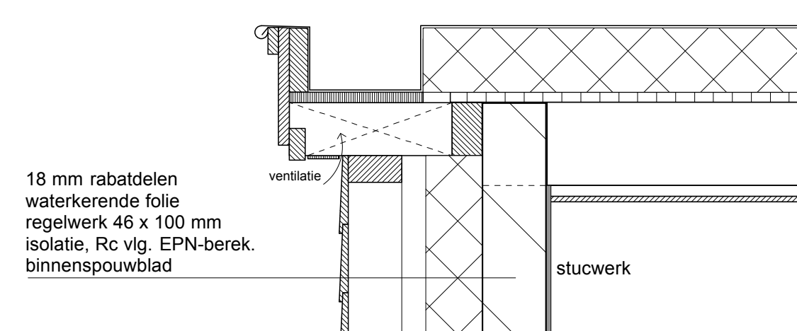
dakranddetail bijkeuken
