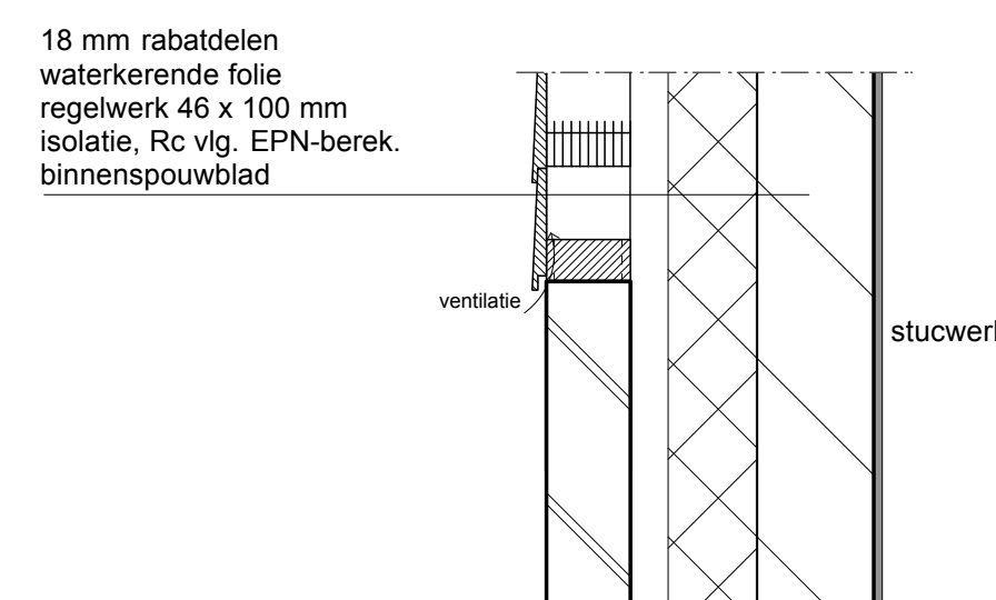
overgang houten gevel/ trasraam
