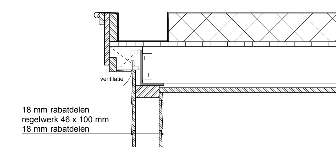
dakranddetail luifel met gevel
