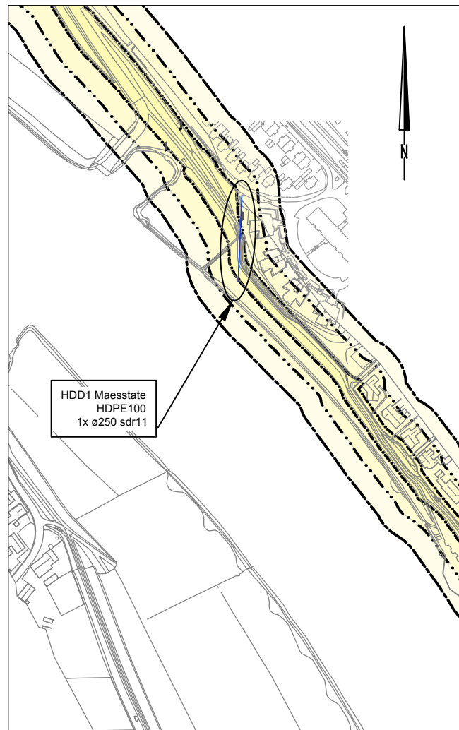
Situatieoverzicht Schaal 1:5000
