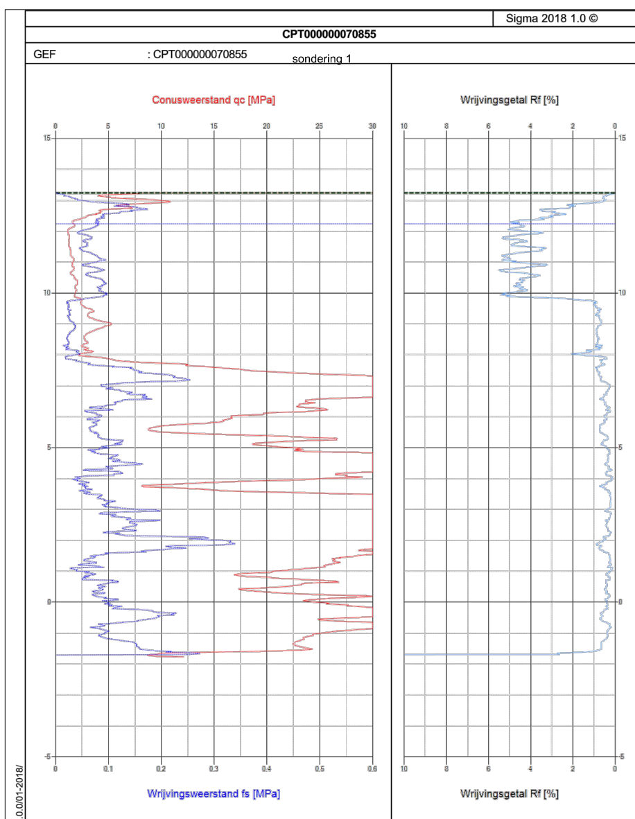
Sondering
