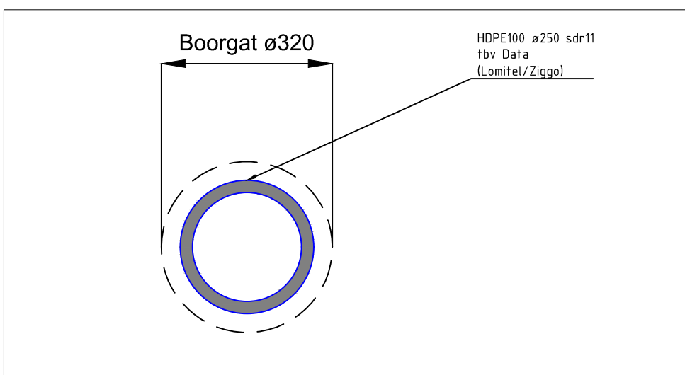
BUNDELDOORSNEDE Schaal 1:50
