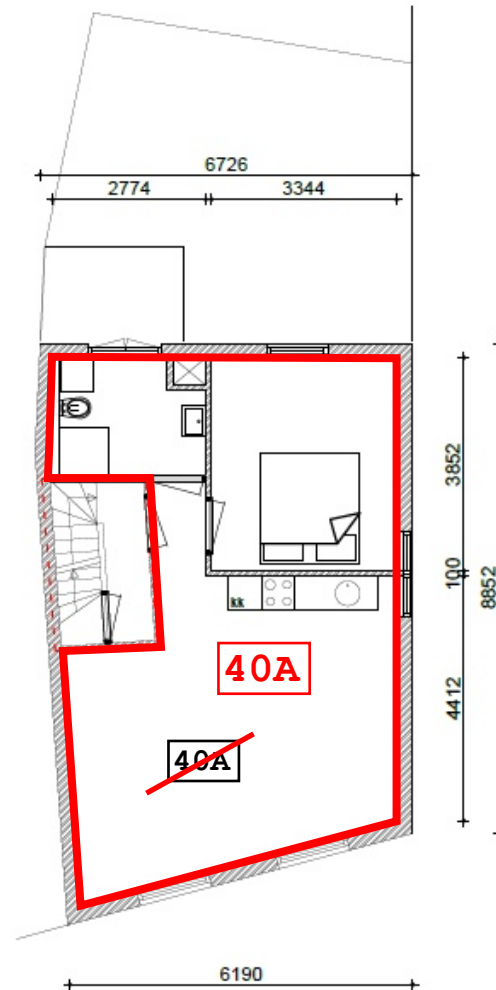
Eerste verdieping
