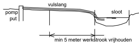
Bestaande Situatie
