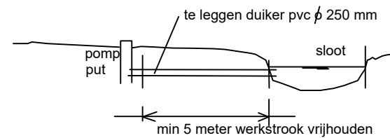
Nieuwe Situatie
