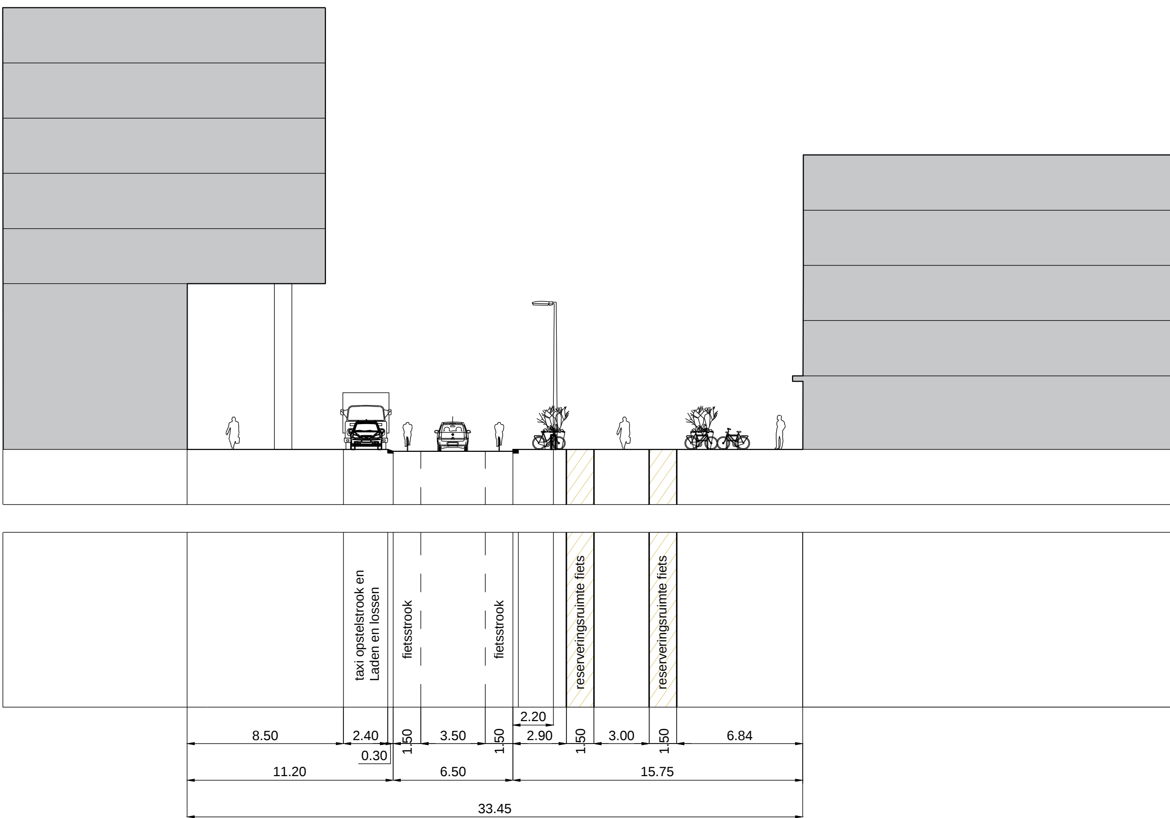
Doorsnede A-A' Schaal- 1:200
