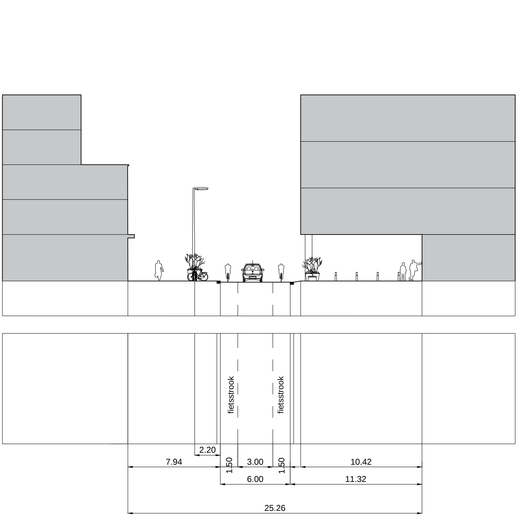
Doorsnede C-C' Schaal- 1:200
