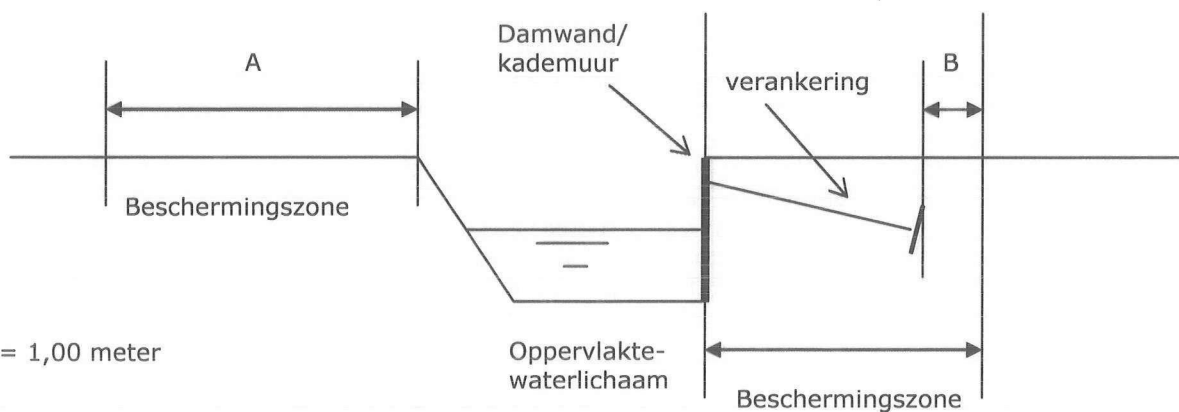
Principeprofiel verankerde damwand of kademuur:
