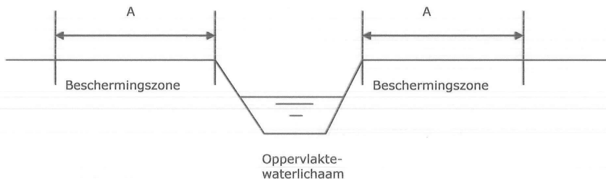
Principeprofiel accoladeprofiel:
