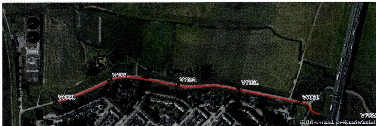
Figuur 3.5: Locatie piping/stabiliteitsscherm (rode lijn) in het binnentalud
