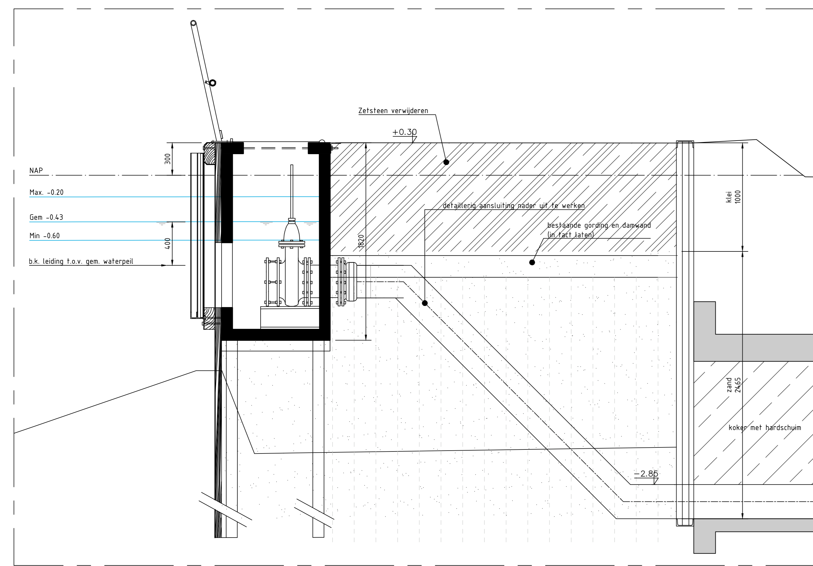
DOORSNEDE SITUATIE schaal: 1:20
