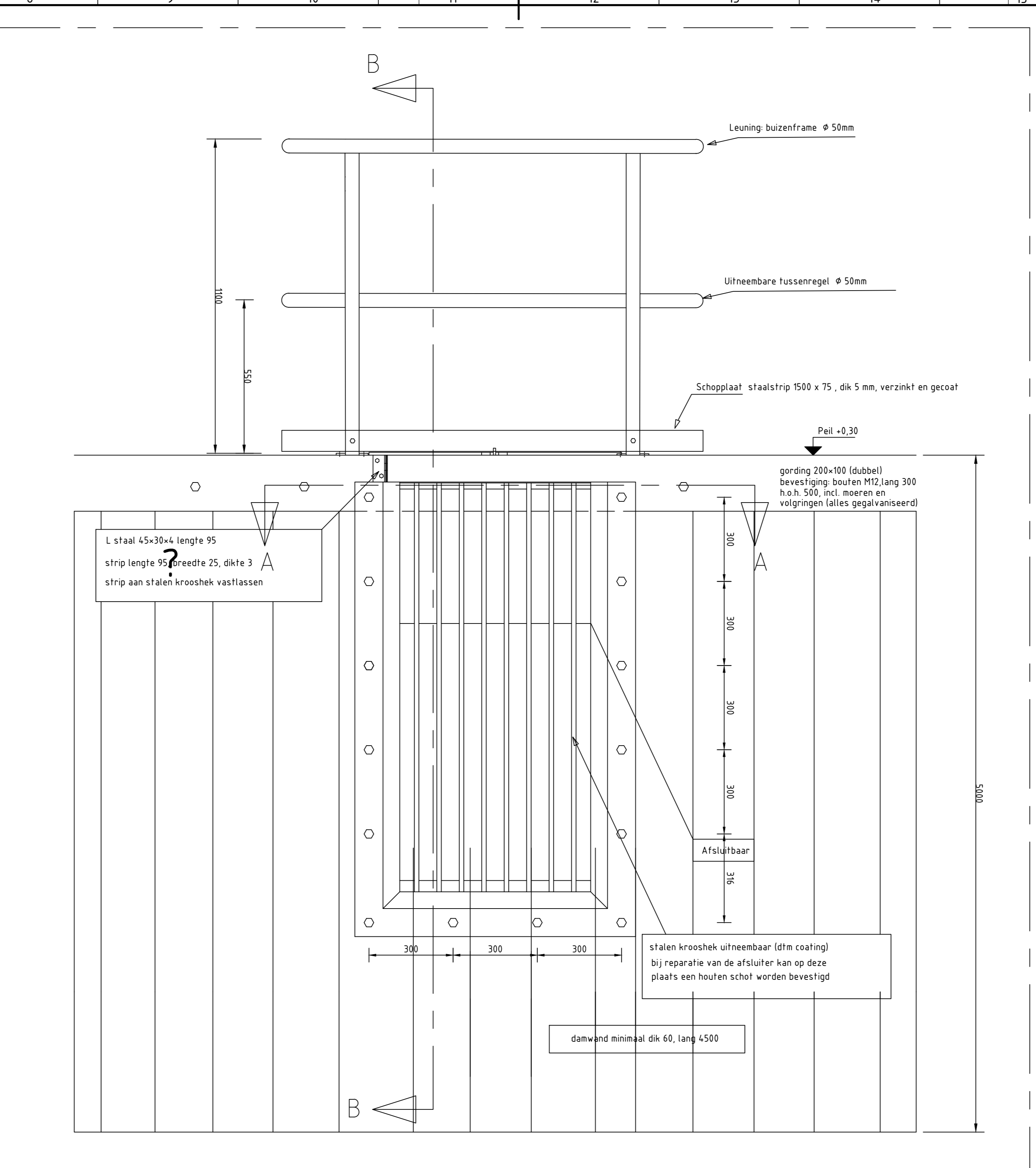
VOORAANZICHT schaal: 1:10
