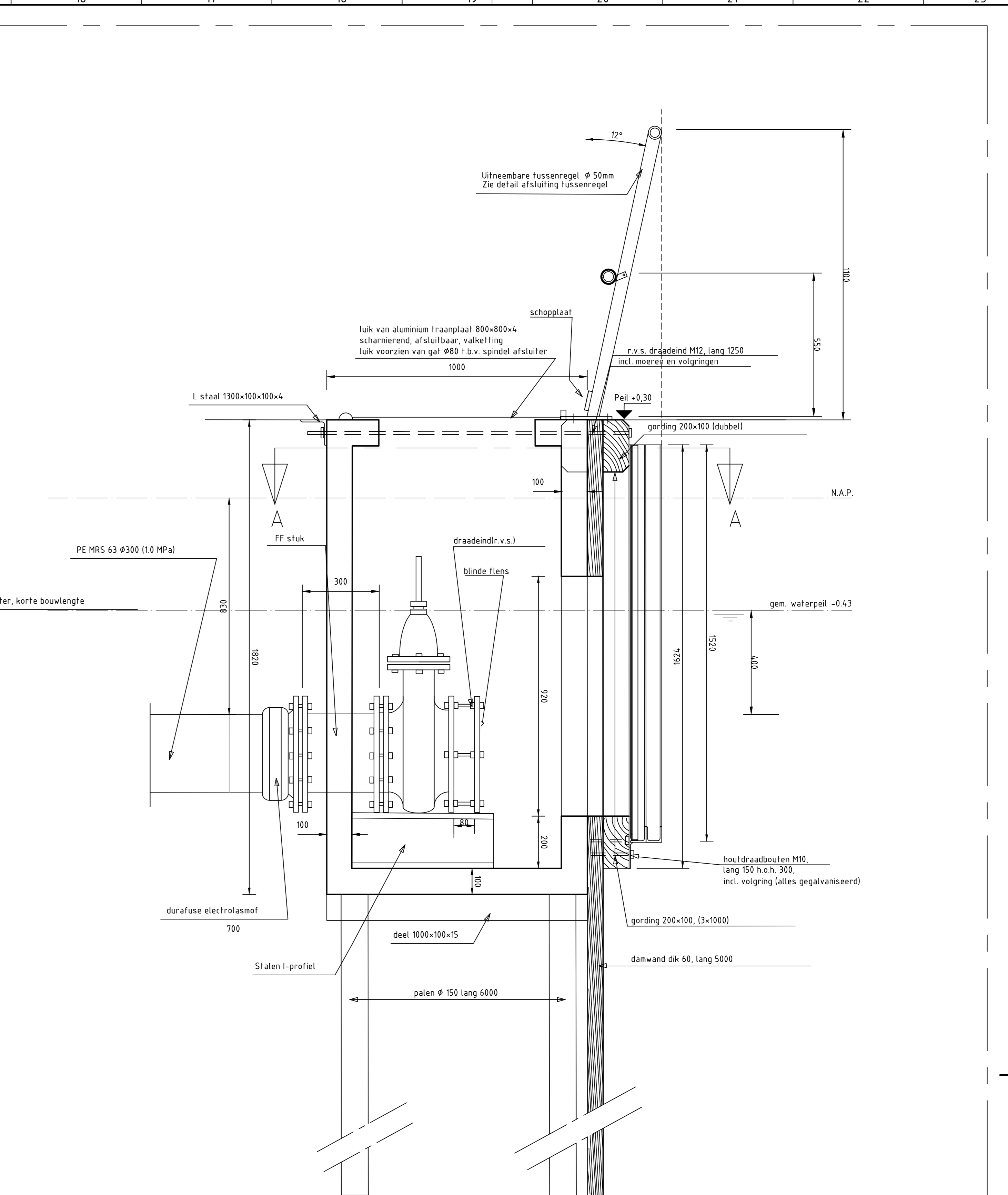
DOORSNEDE B-B schaal: 1:10
