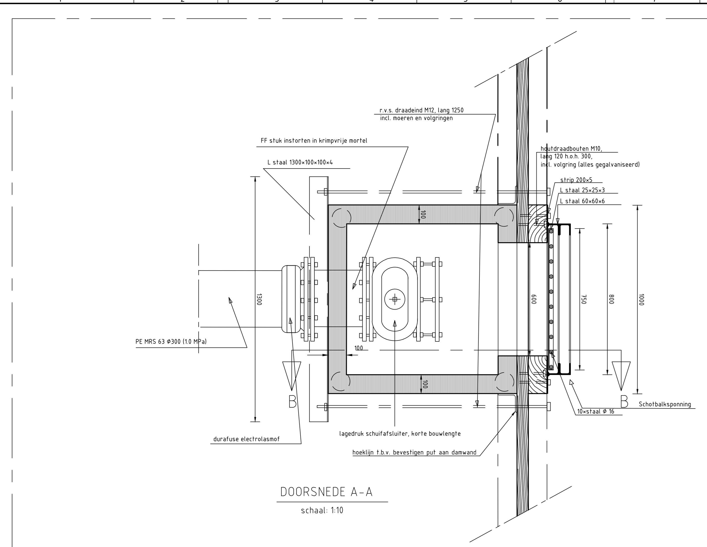
DOORSNEDE A-A schaal: 1:10
