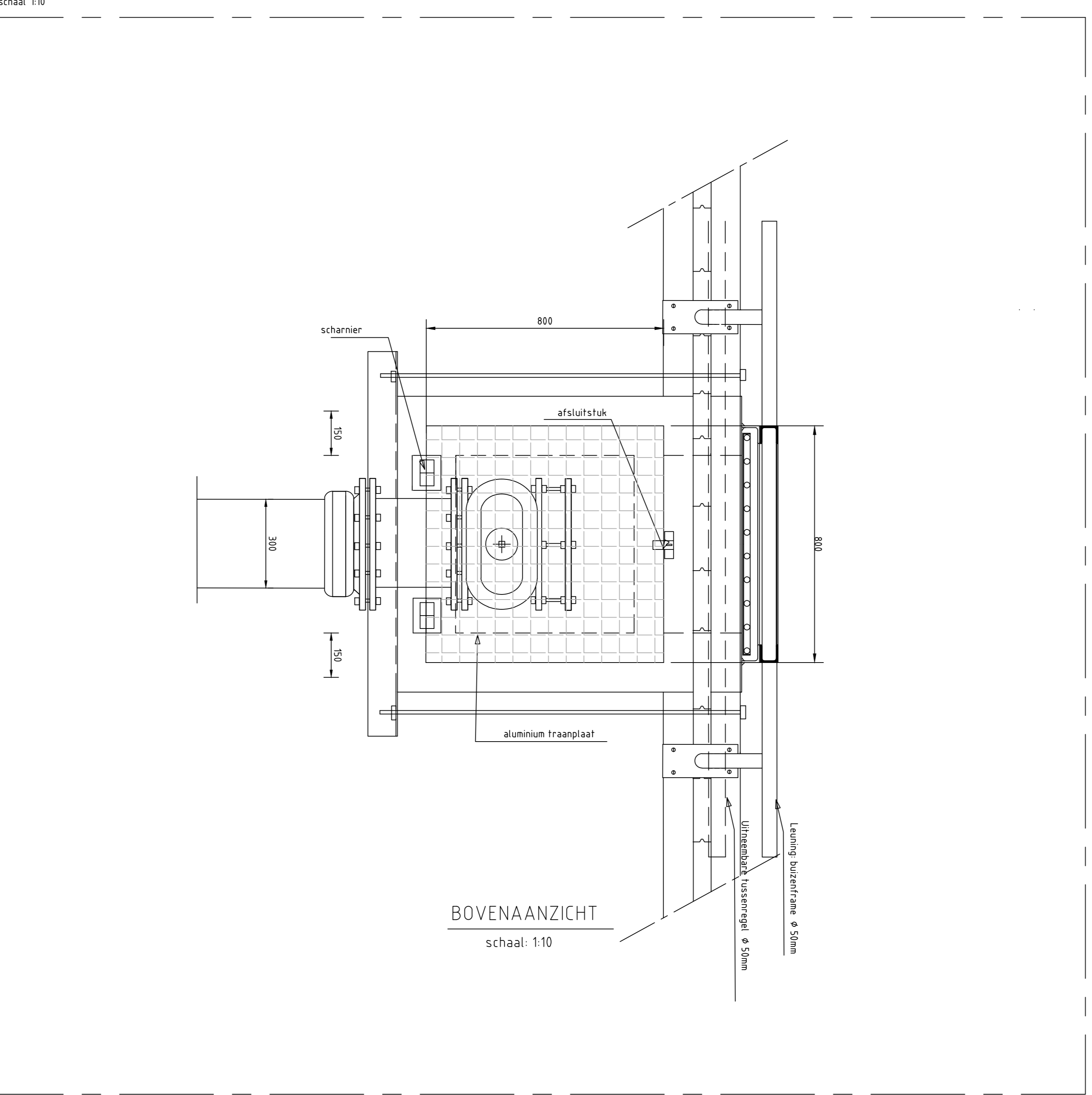
BOVENAANZICHT PUT schaal: 1:10
