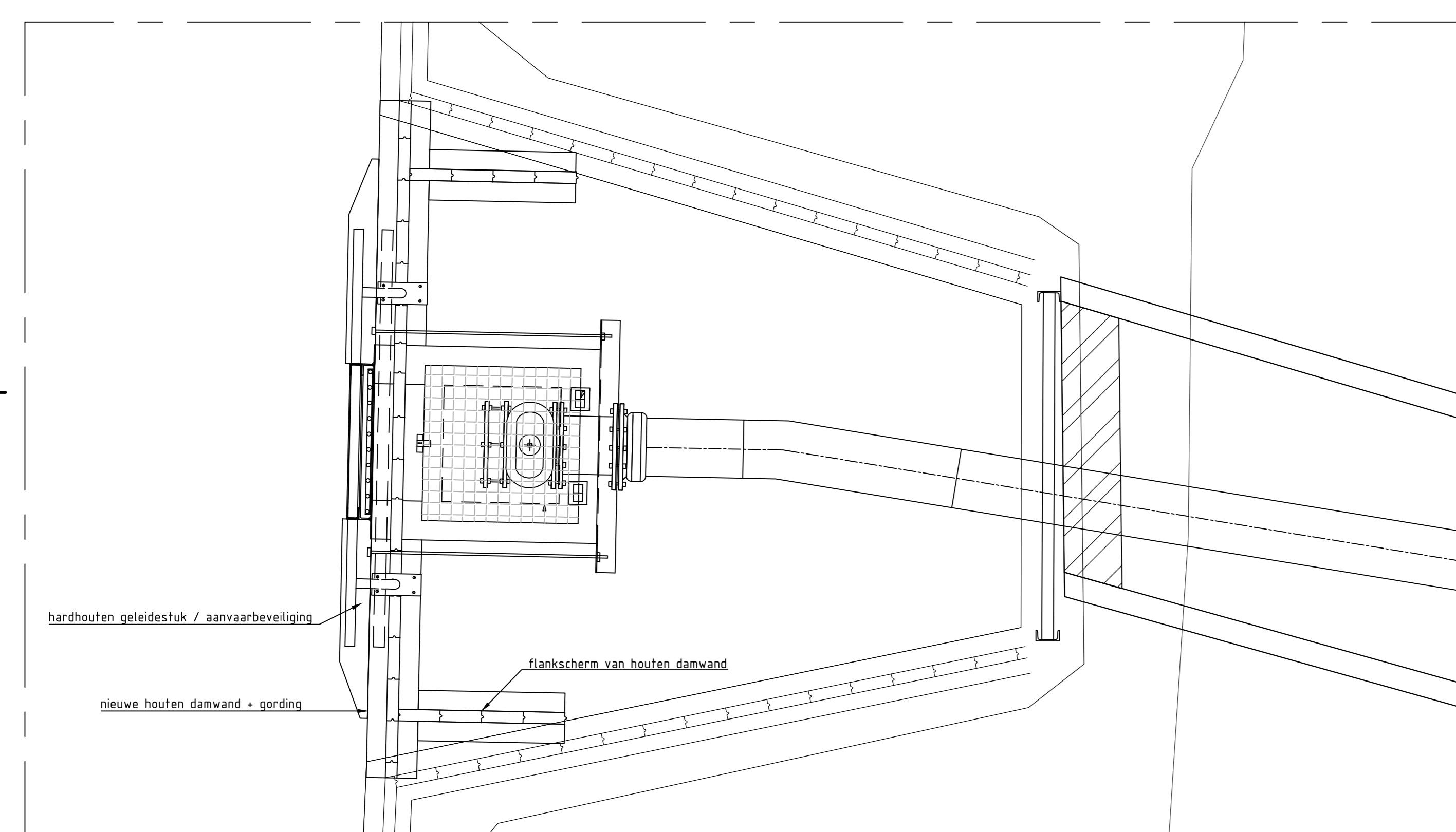
BOVENAANZICHT SITUATIE schaal: 1:20
