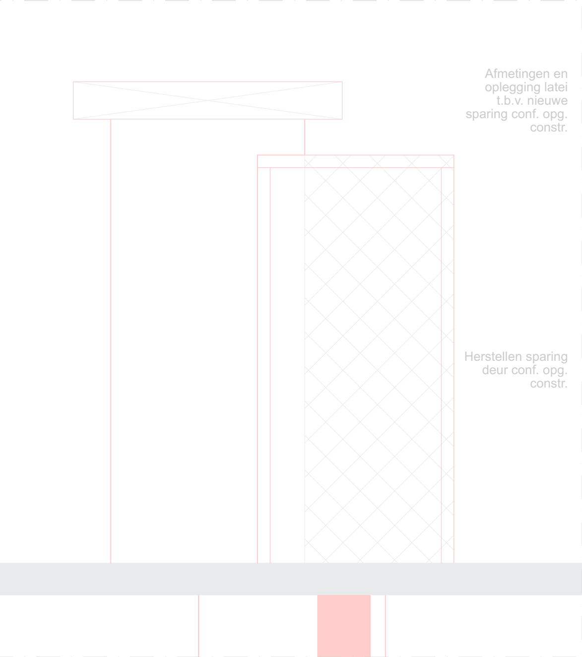
INTERIEURFRAGMENTA 1:20 (principe hoe sparring vorm te geven t.b.v. inleggen nieuwe latei conf. opg. constr.)
