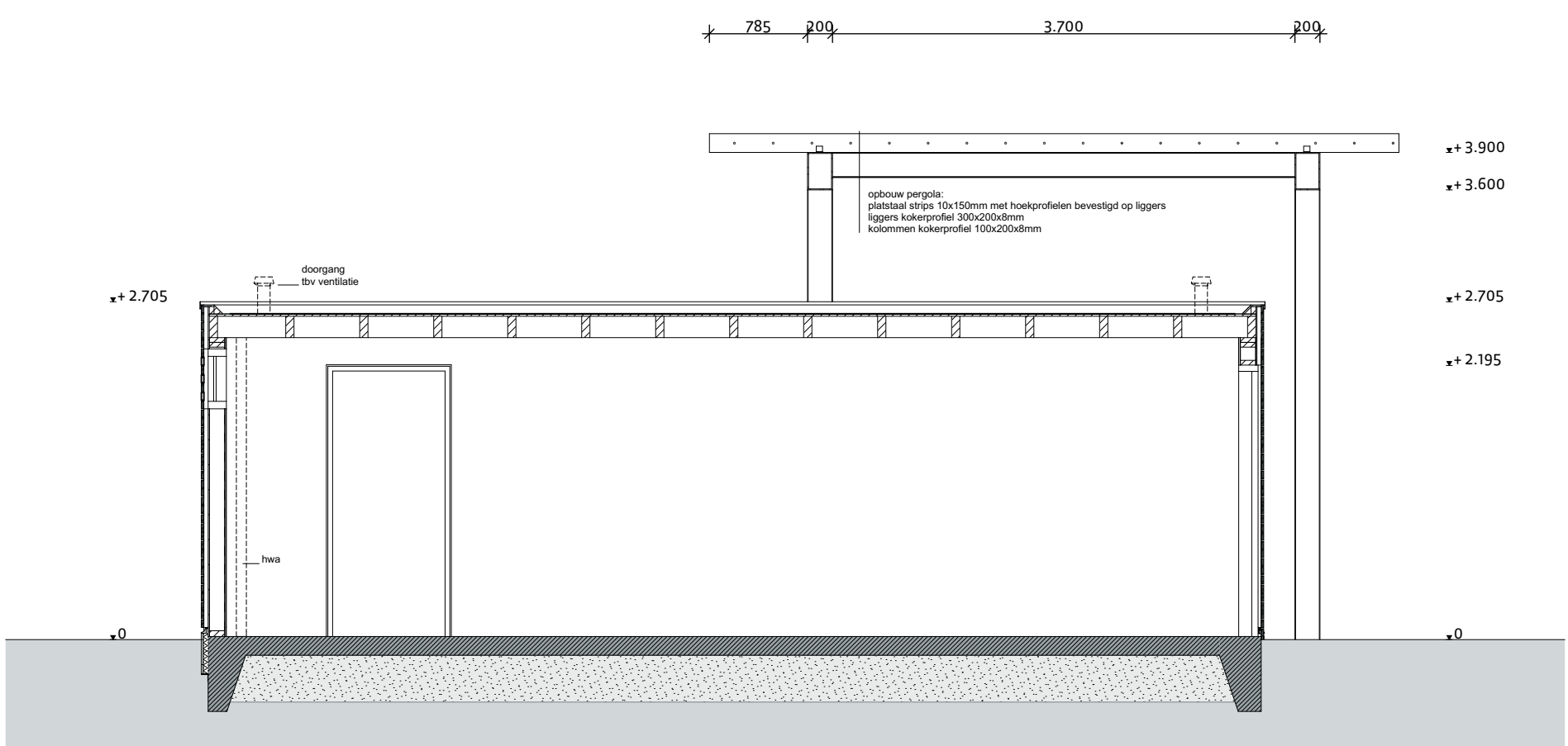
Doorsnede D-D
