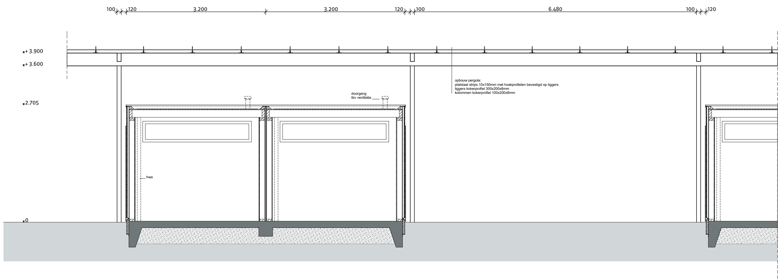
Doorsnede C-C
