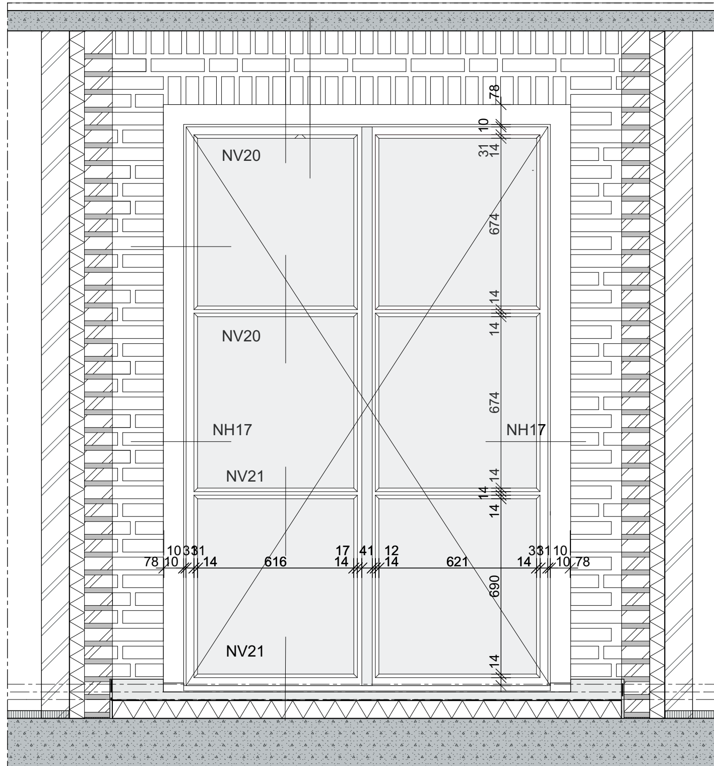
Loggia aanzicht nieuw - renovatie kozijn Woning G04
