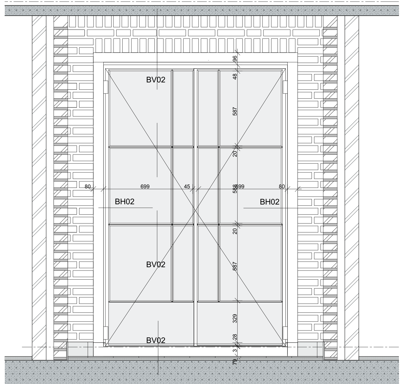
Stalen pui loggia woning G04 demonteren voor hergebruik
