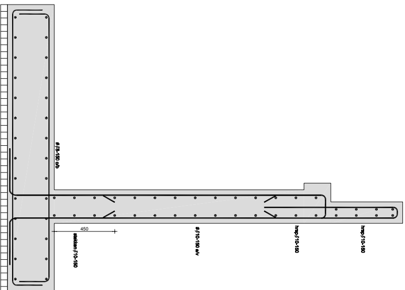
PRINCIPE DETAIL 11 wapening nieuwe keervand
