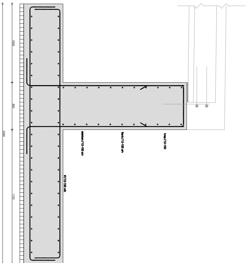
PRINCIPE DETAIL 7 wapening nieuw lathoofd
