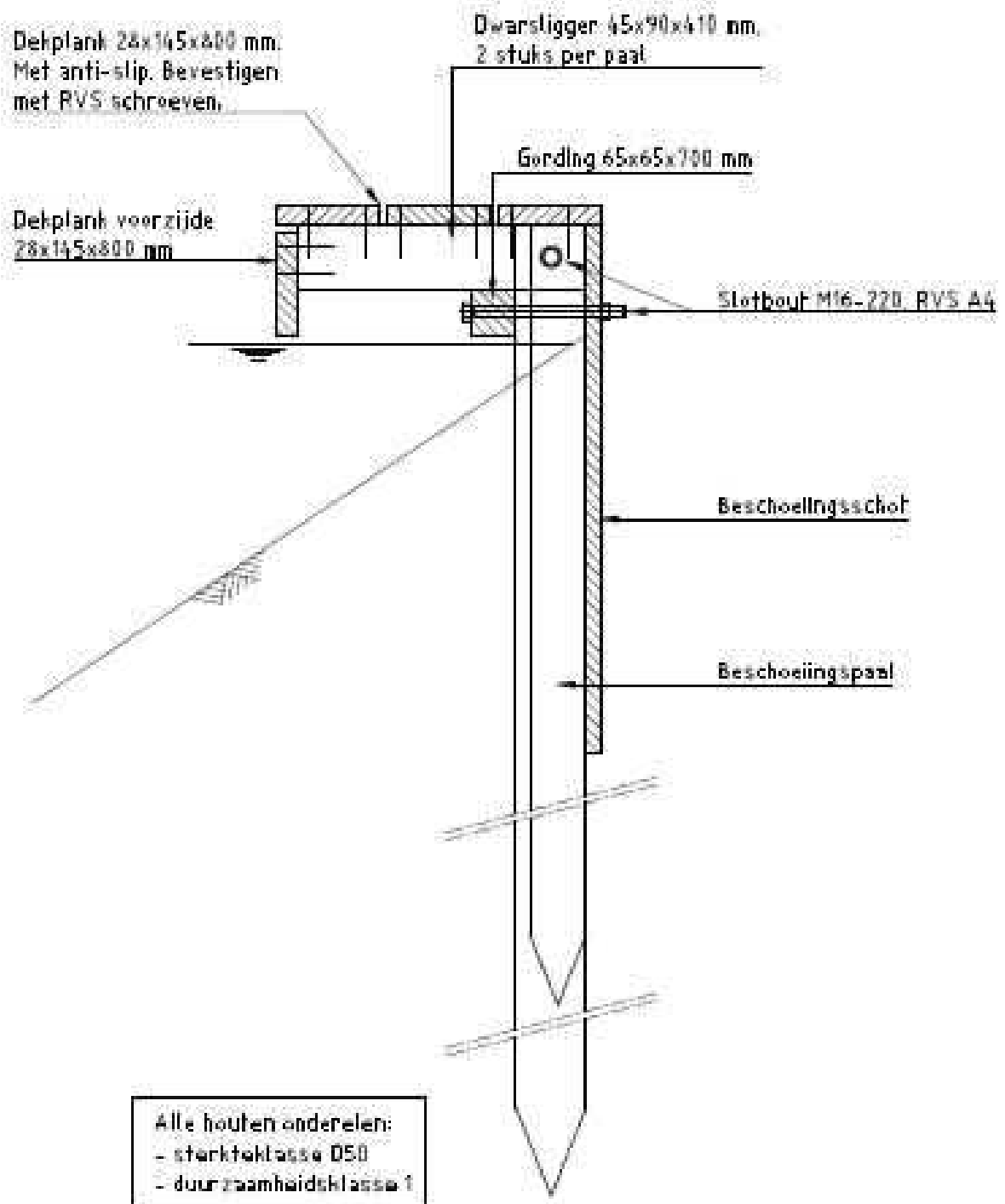
Doorsnede principe oplossing opstapplaatsen Schaal 3:10
