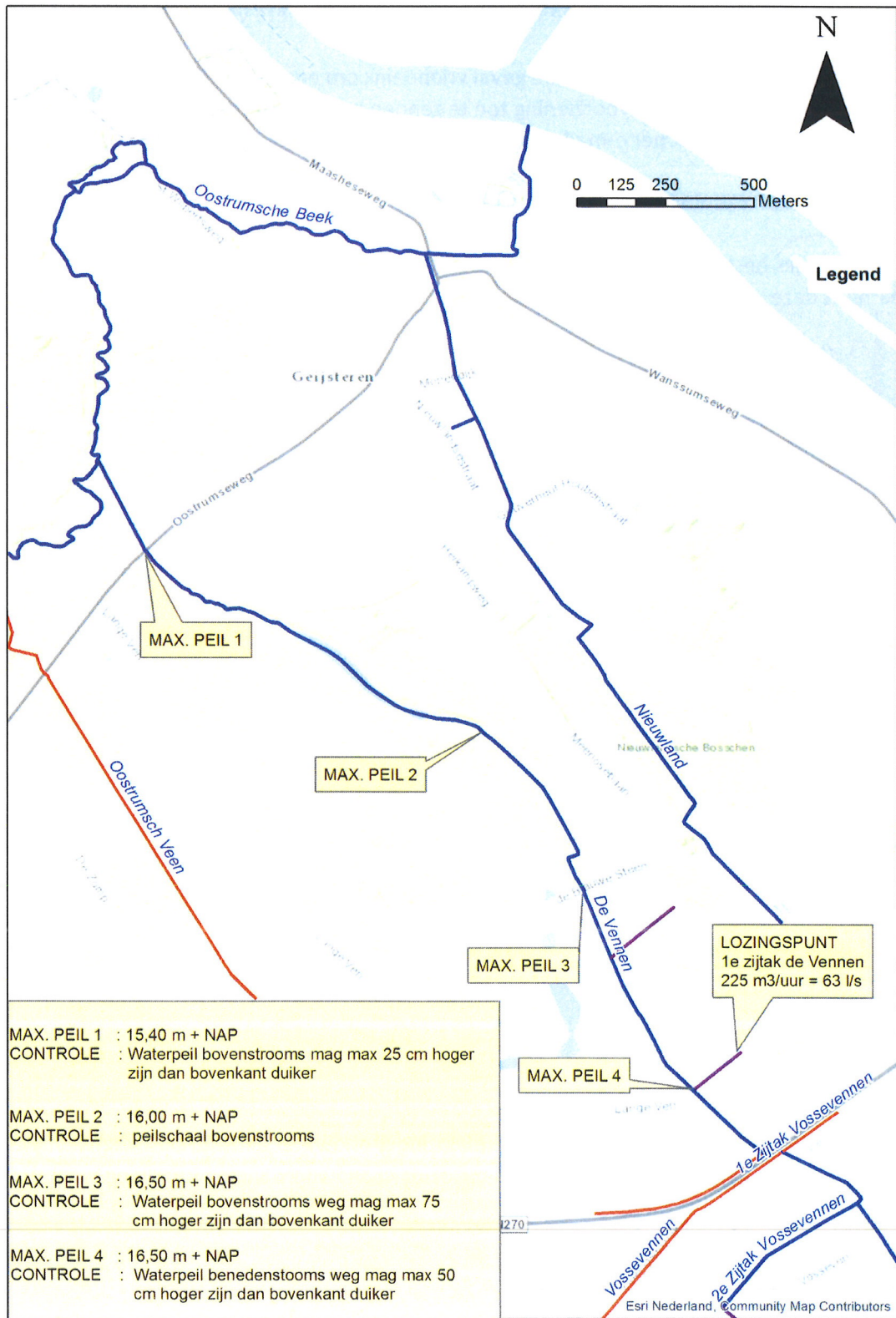
Bijlage 1: maximale peilen De Vennen bij lozing grondwater aanleg Rondweg-west Wanssum
