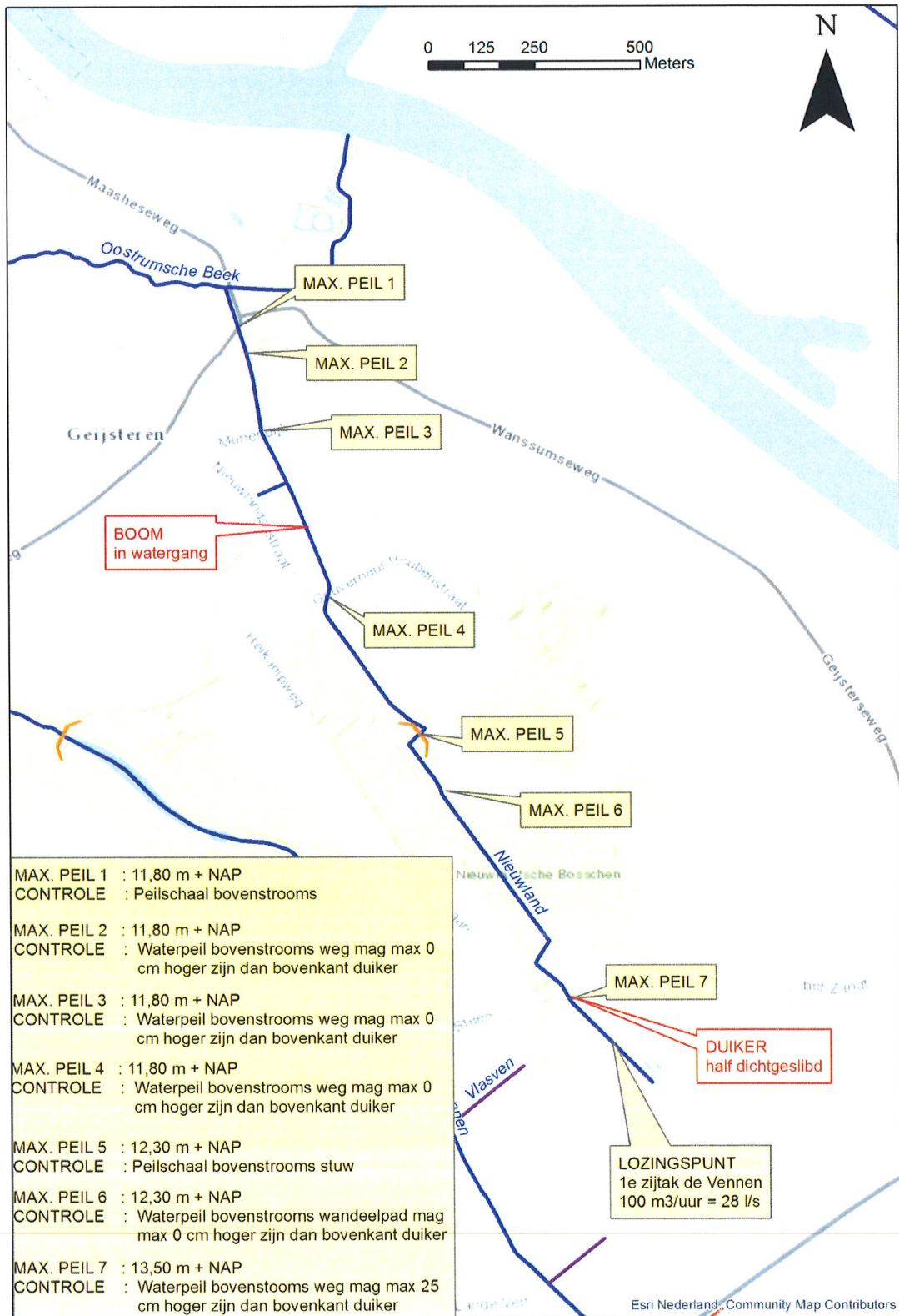
Bijlage 2: maximale peilen Nieuwland bij lozing grondwater aanleg Rondweg-west Wanssum
