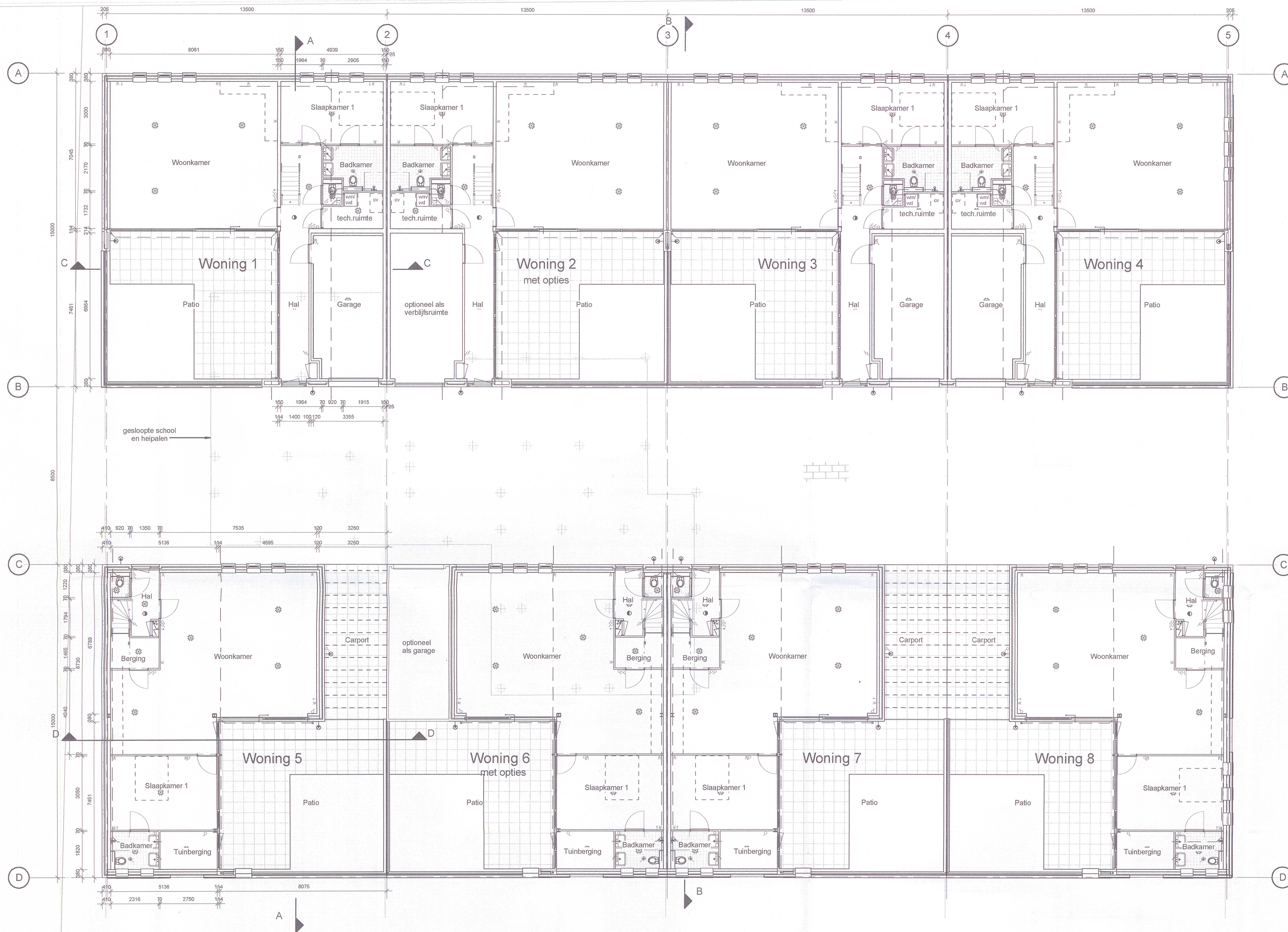
Begane Grond
