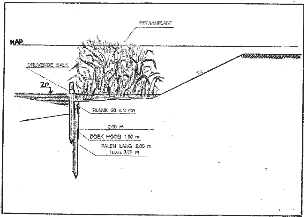
Bijlage 6: "technische natuurvriendelijke oevers".
