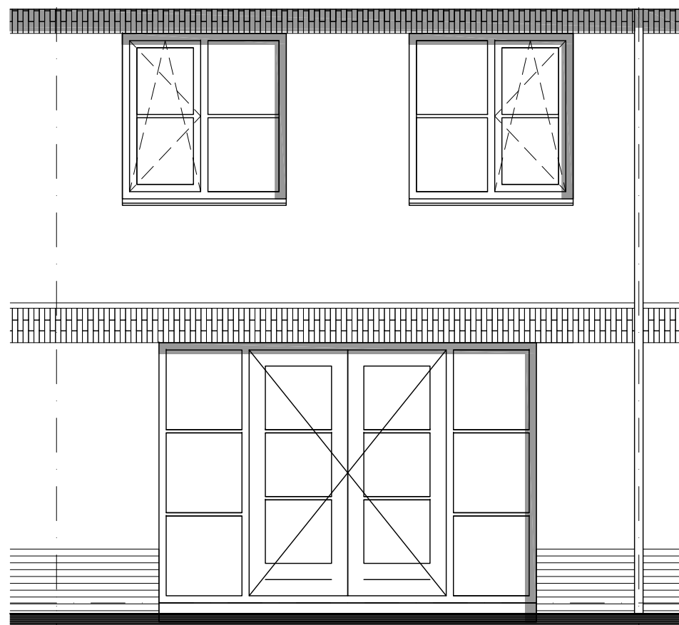
achtergevel
