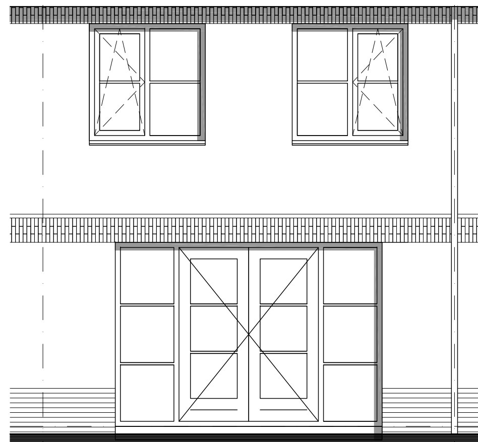
achtergevel
