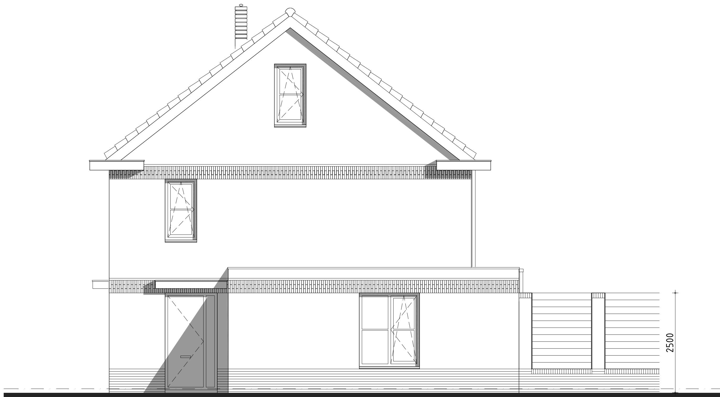
rechter zijgevel
