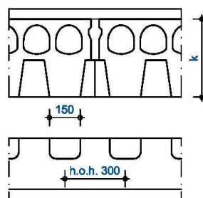
AANZICHTEN RANDOPLEGGING
