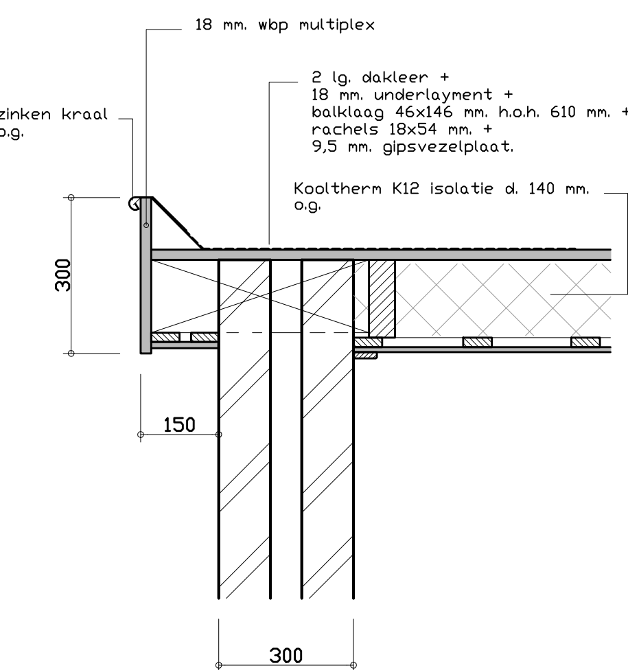
DETAIL 4. schaal 1:10.
