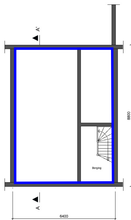
Kelder (nieuw)
