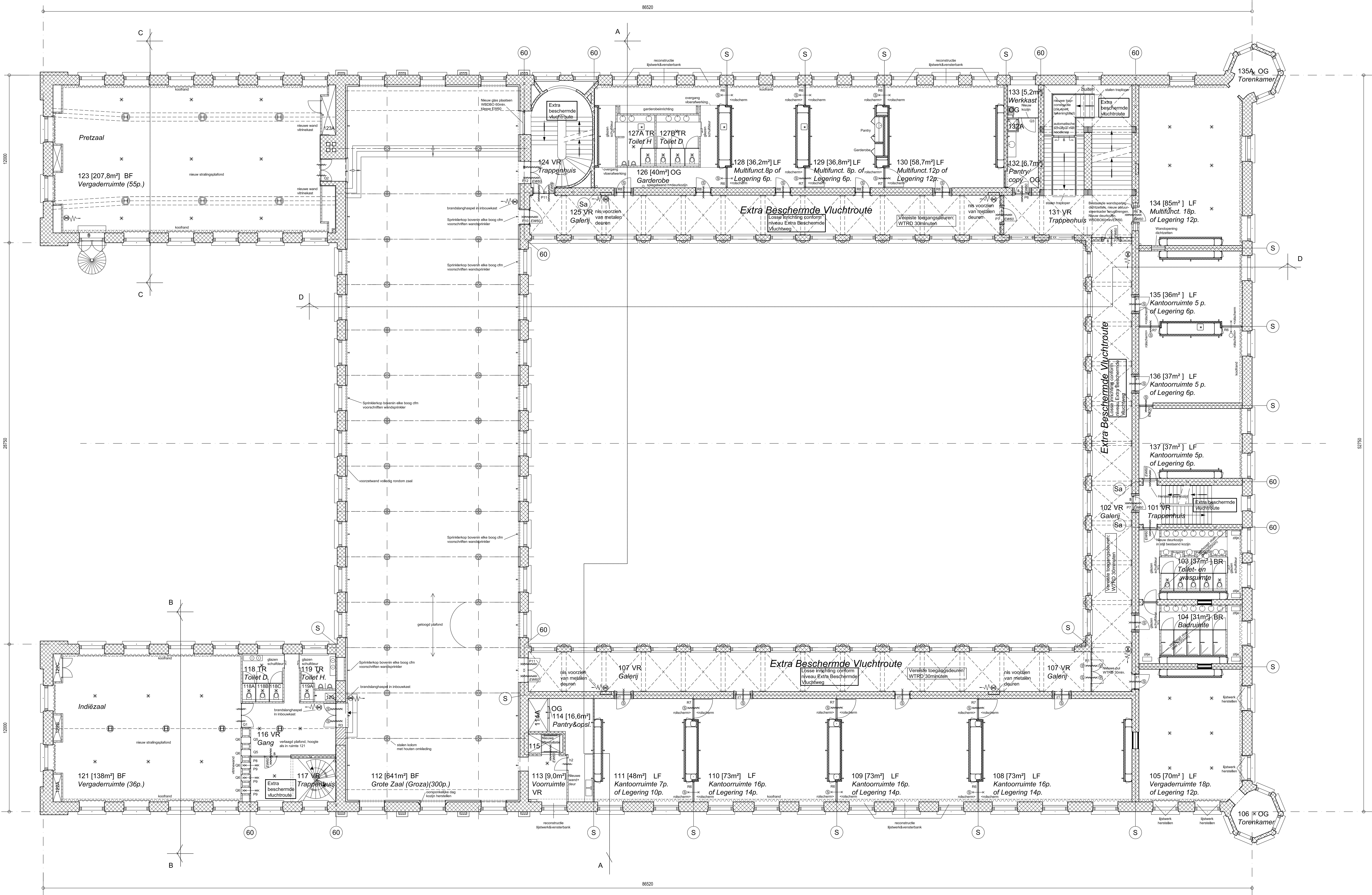
Eerste Verdieping
