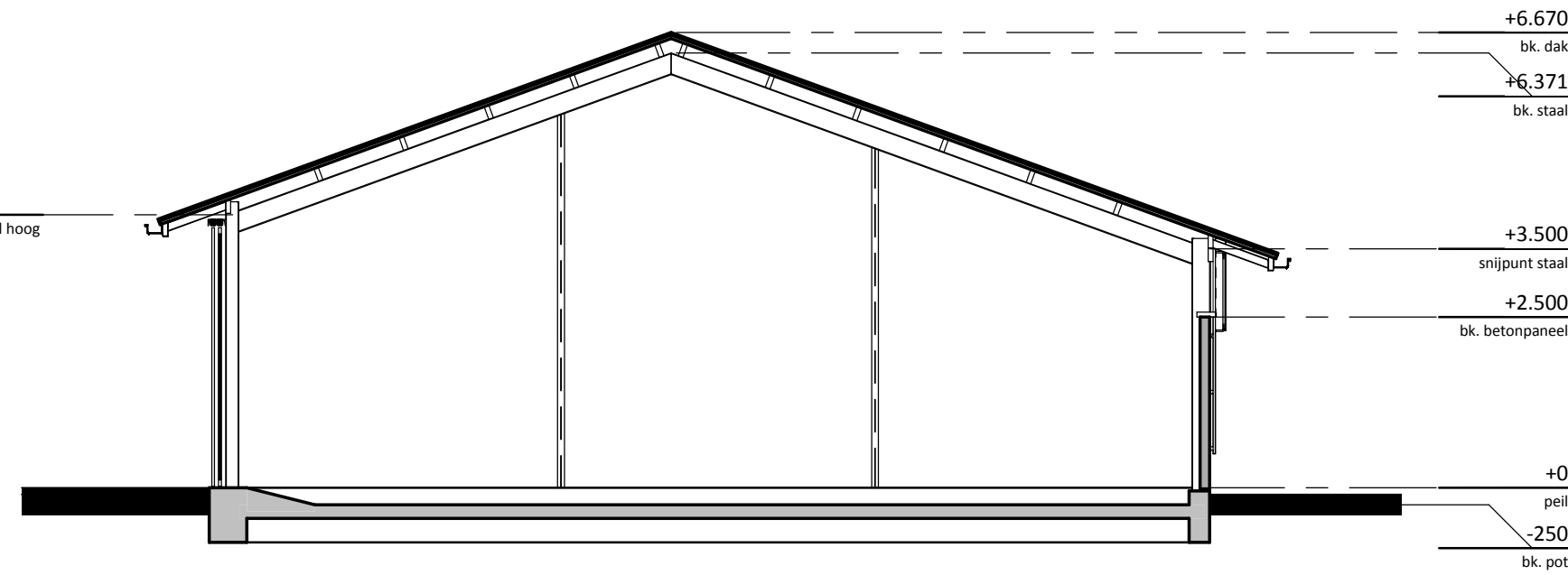
doorsnede B
