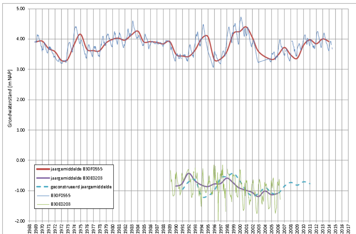
Figuur I-8 Gemeten en gemodelleerde freatische grondwaterstanden in de Kokshoornpolder en een meetpunt in Noordwijk (bron:DINoloket.nl)
