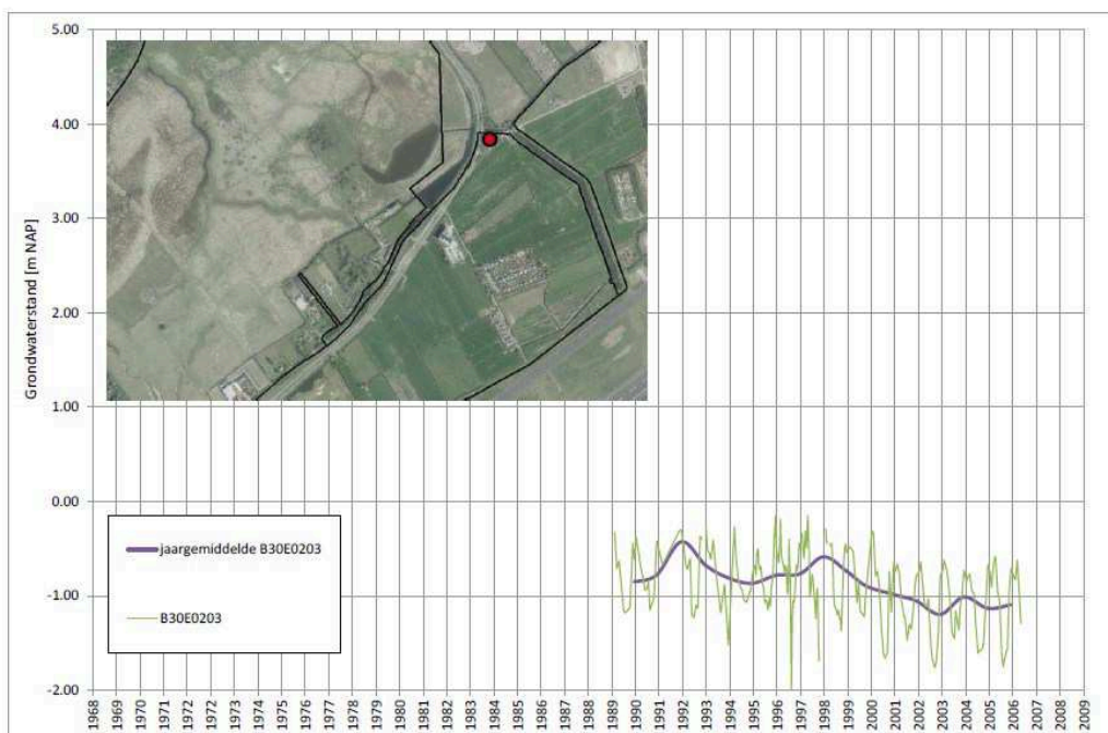
Figuur I-7 Locatie peilbuis (B30E0203) en gemeten freatische grondwaterstanden (bron: DINoloket.nl)
