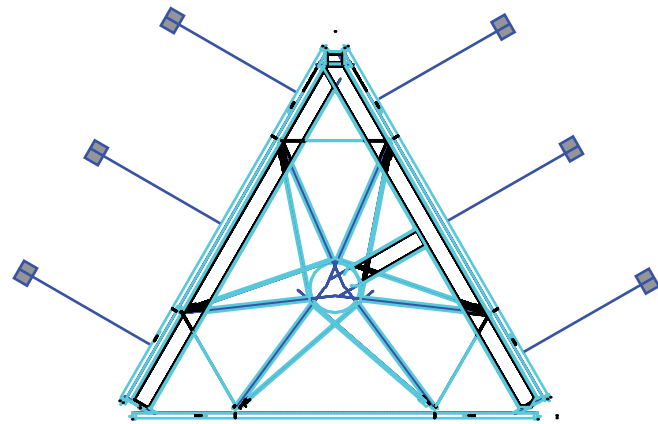
BOVENAANZICHT (BESTAAND)
