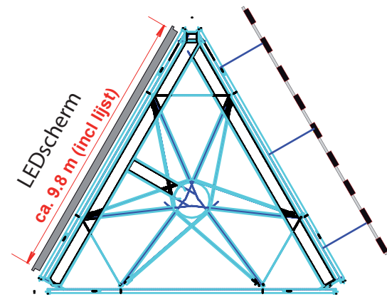
BOVENAANZICHT (NIEUW)
