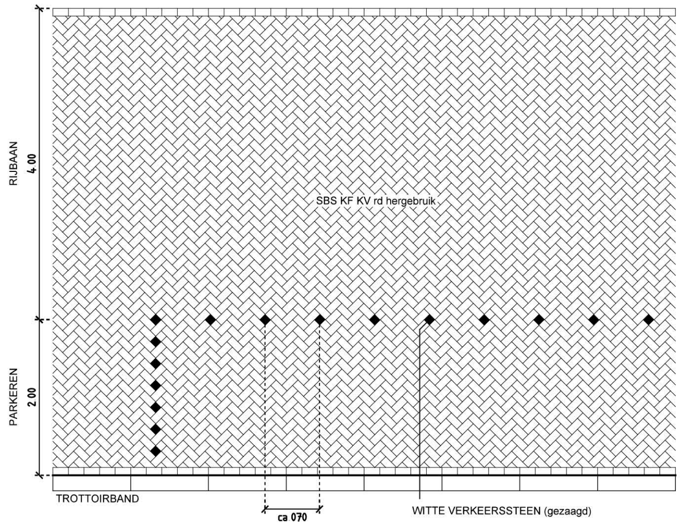
DETAIL PARKEERMARKEERING schaal 1:50
