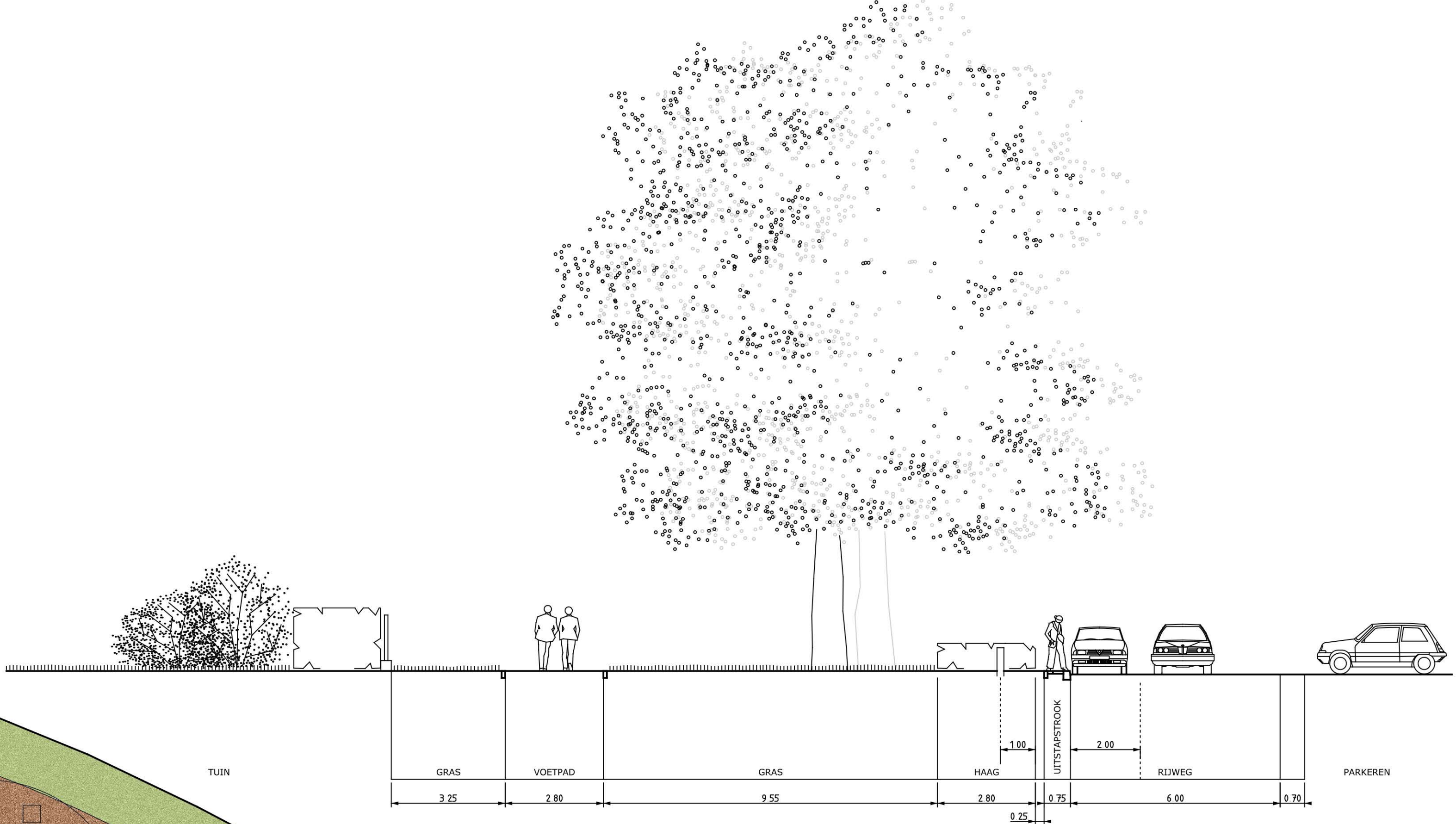
DWARSPROFIEL schaal 1:100
