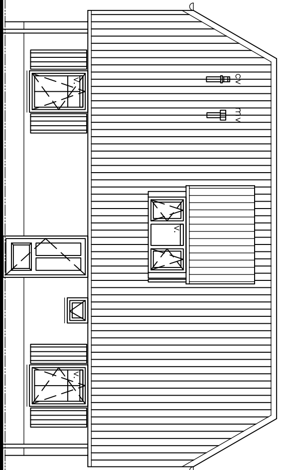
Linkerzijgevel (nieuw)
