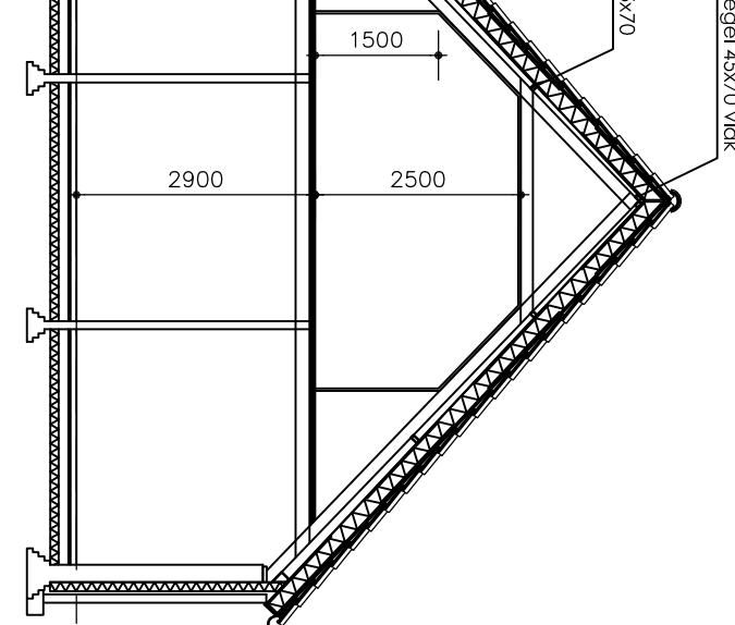
Doorsnede
