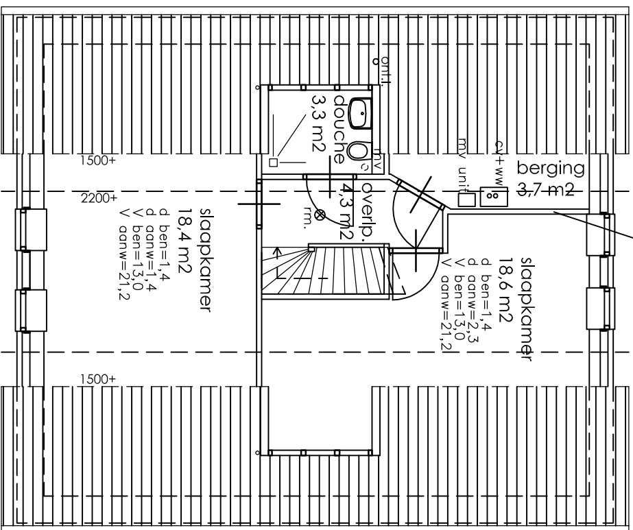
Verdieping (nieuw)
