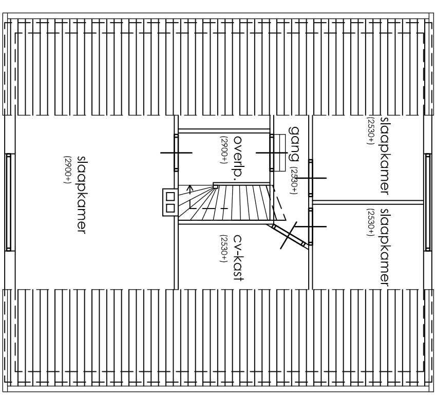
Verdieping (bestaand)
