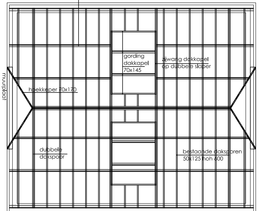
Kappaan
