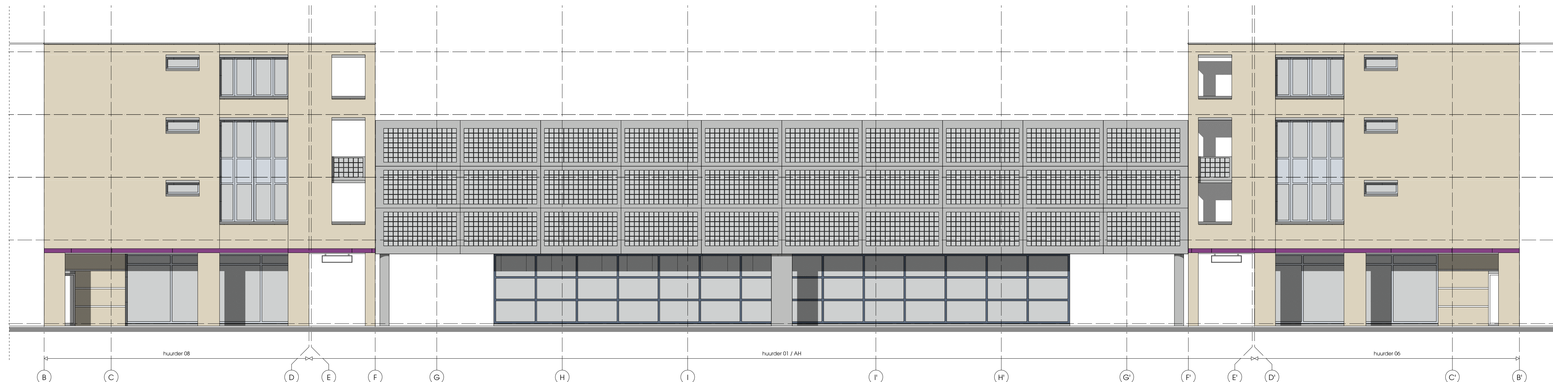
- zuidgevel / B-B -
