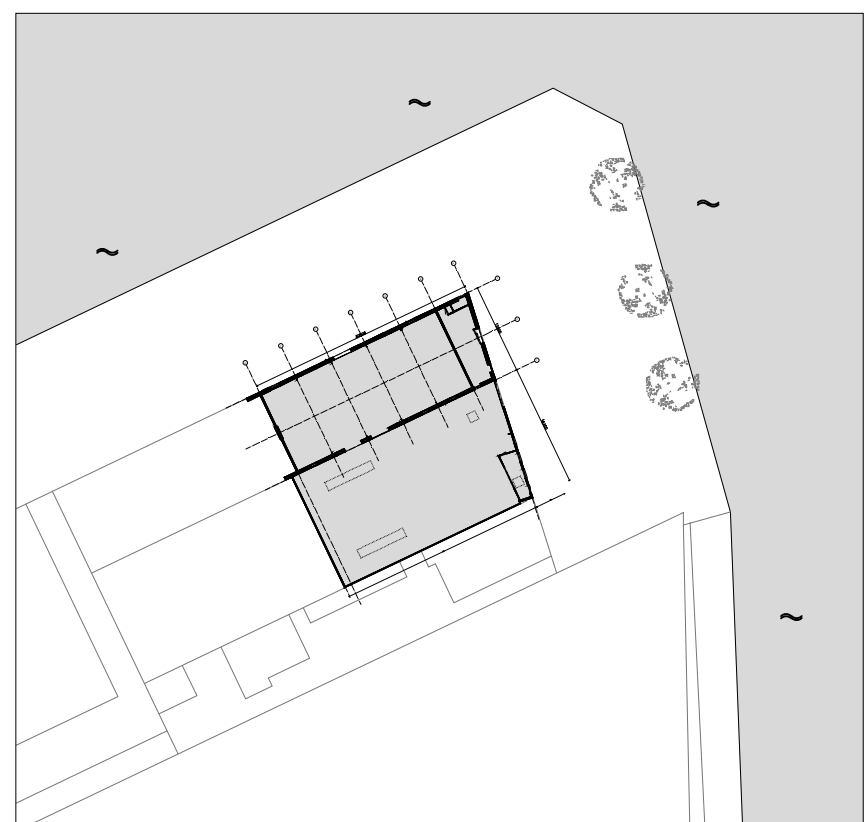
SITUATIE 1:1000
