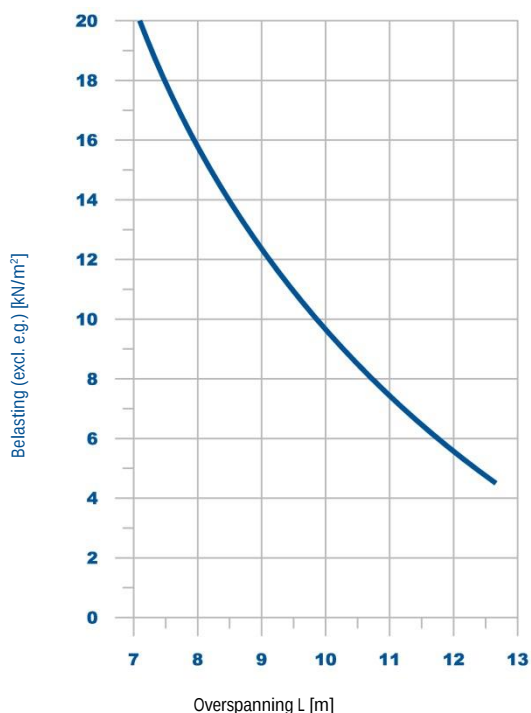
Draagvermogen grafiek
