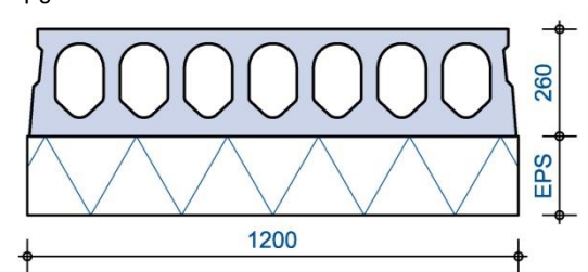
Doorsnede
