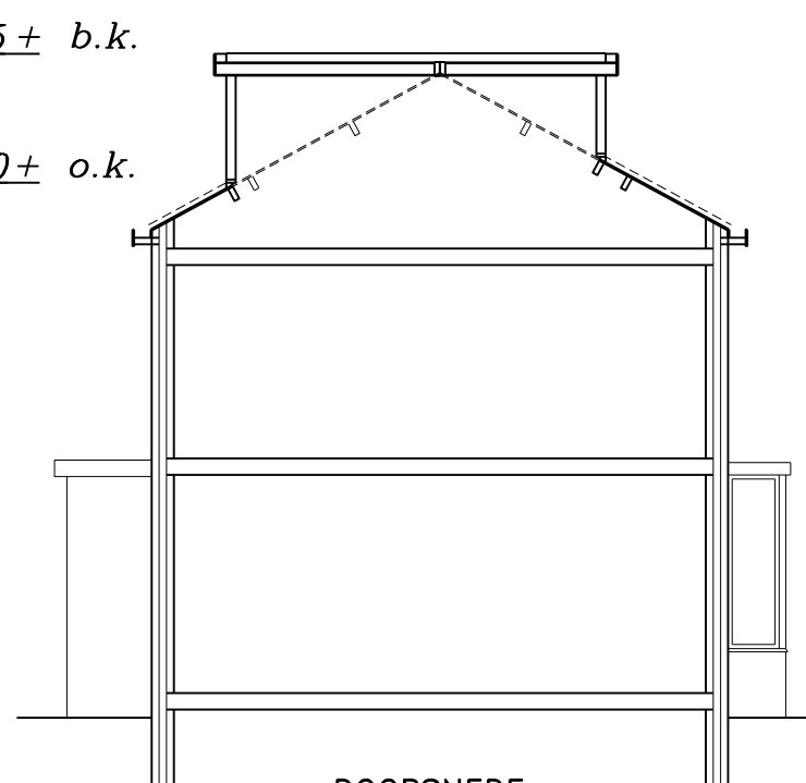
DOORSNEDE NIEUW
