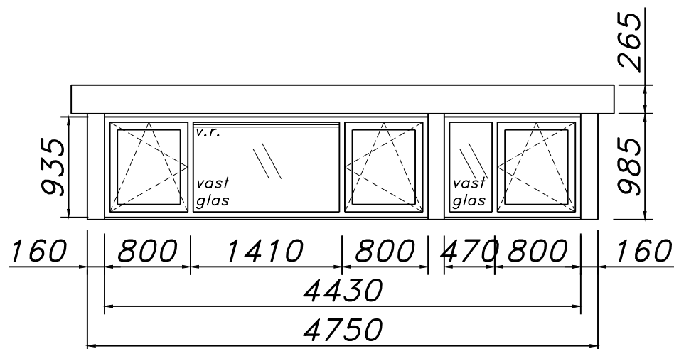
maten in MM. aanzicht dakkapel voorgevel
