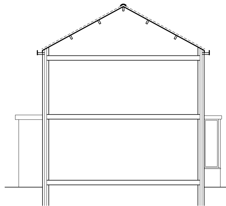
DOORSNEDE BESTAAND
