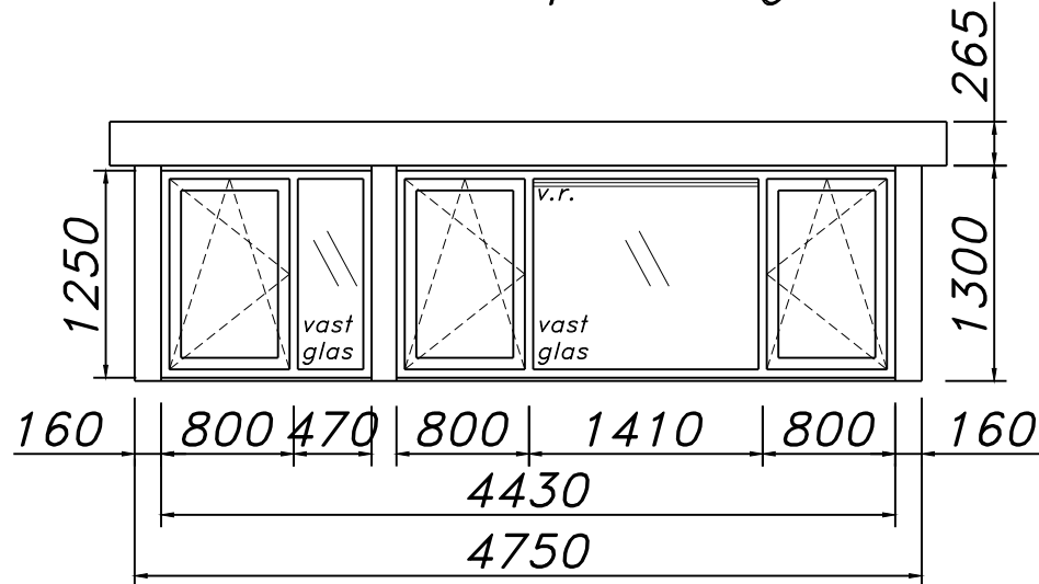
maten in MM. aanzicht dakkapel achtergevel
