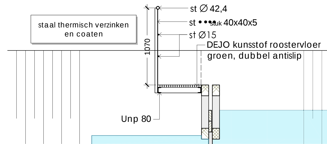
detail bordes met leuning
