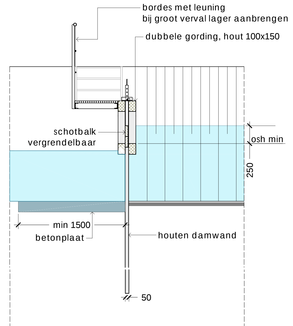
doorsnede a-a
