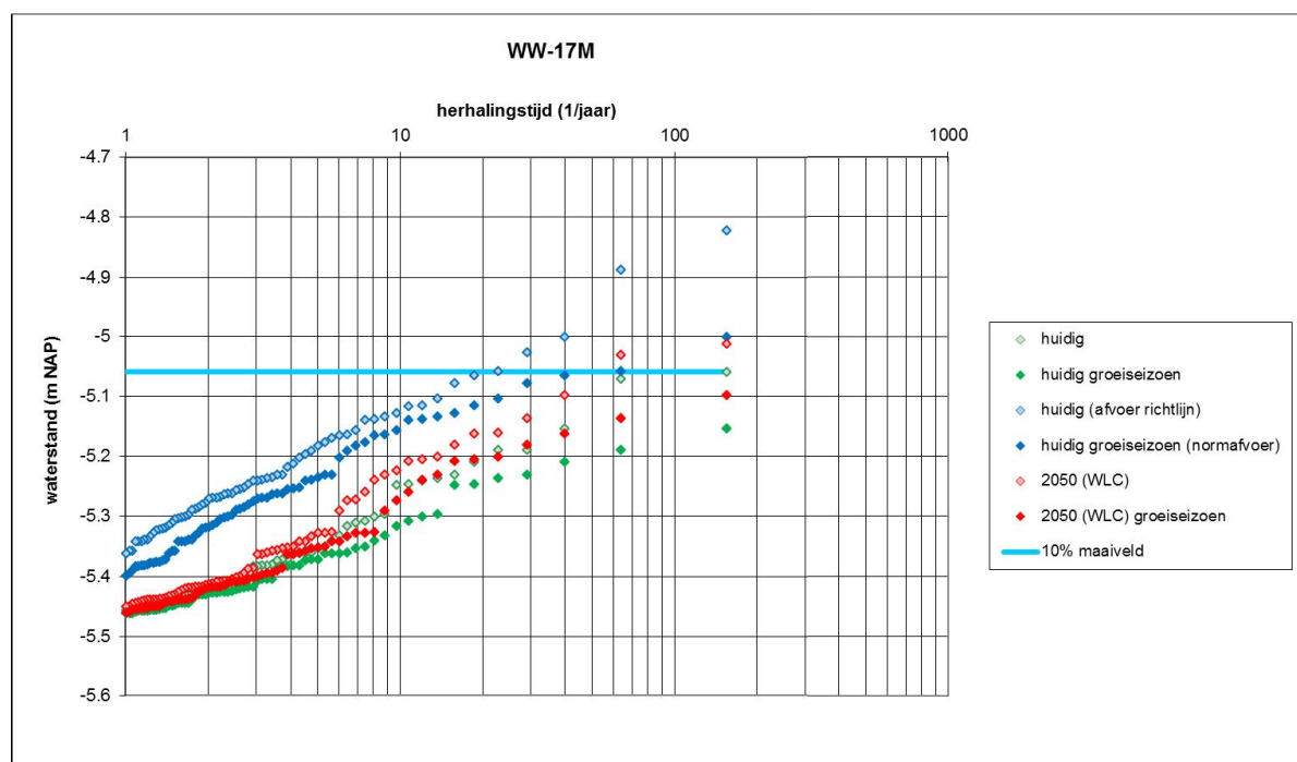
Figuur 4.2: Waterstandkansgrafiek peilvak WW-17M
