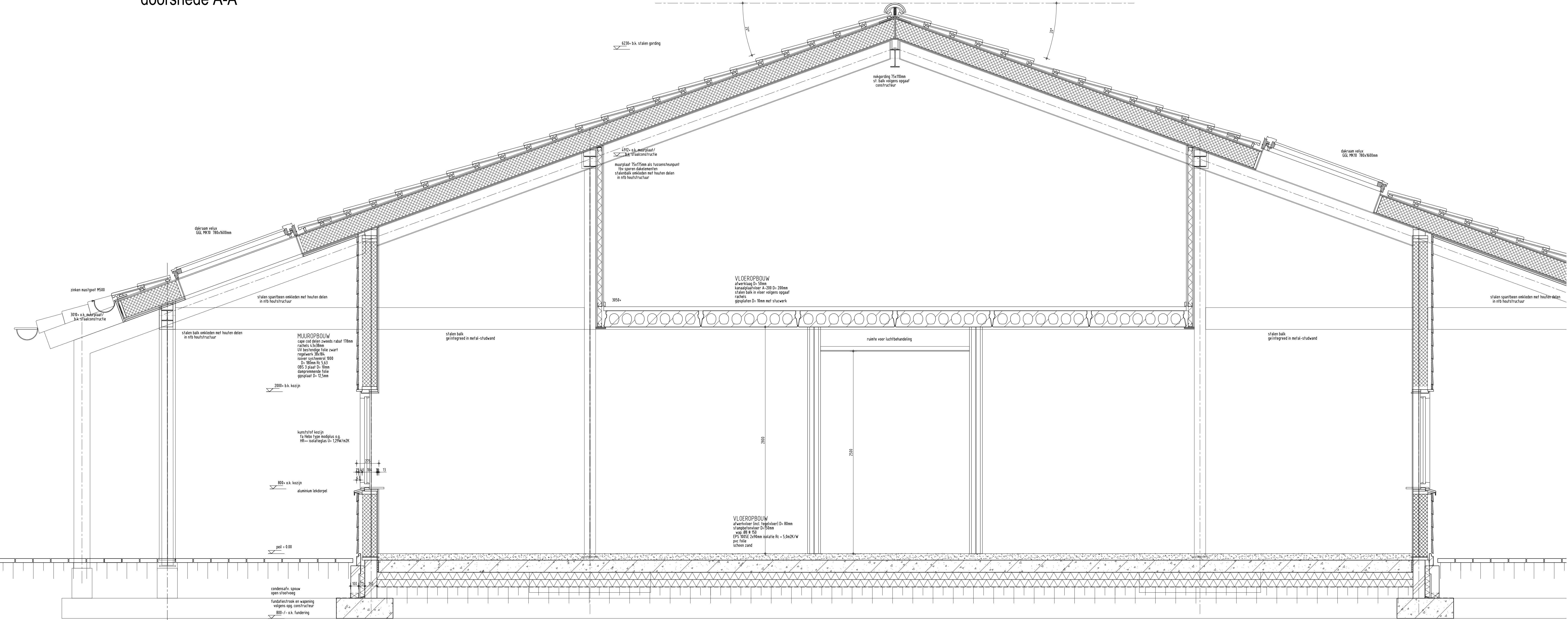
doorsnede C-C
