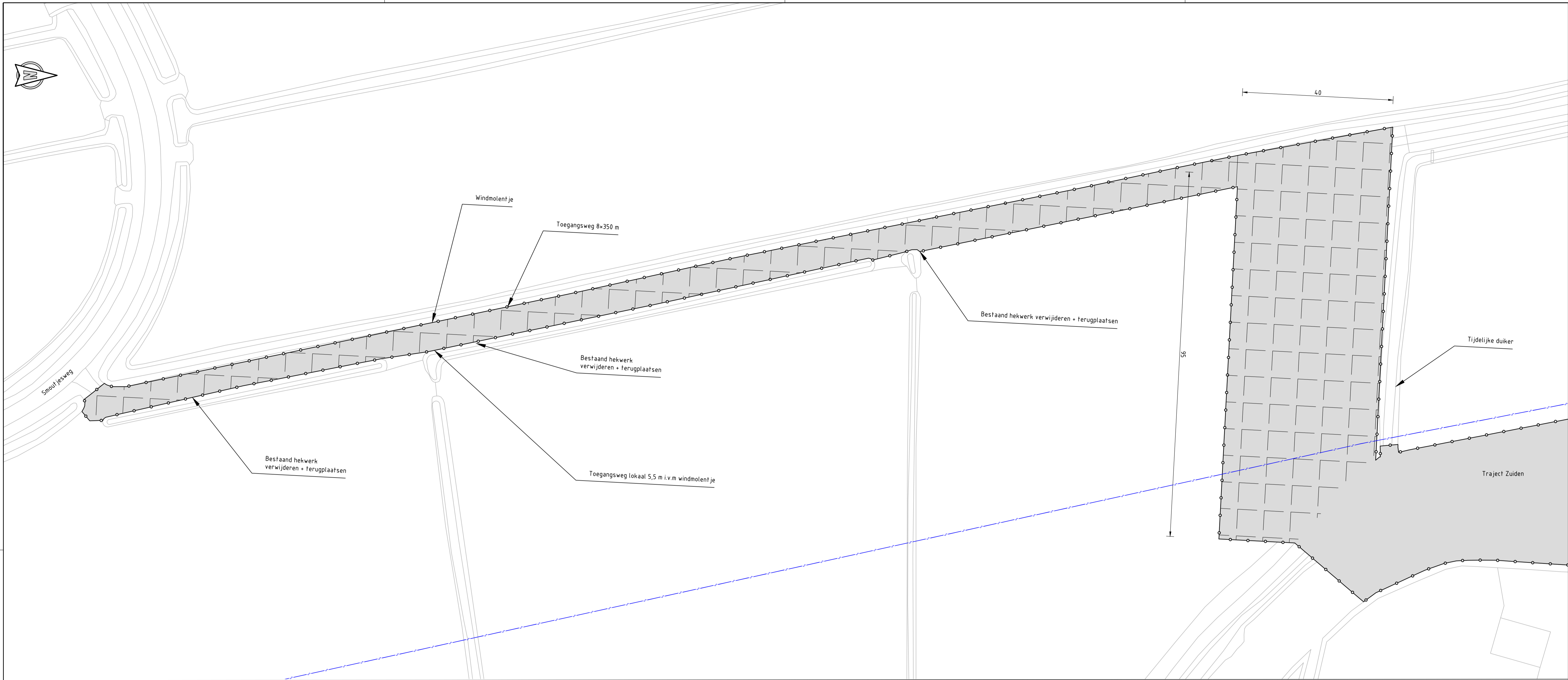
Bovenaanzicht Schaal: 1:500
